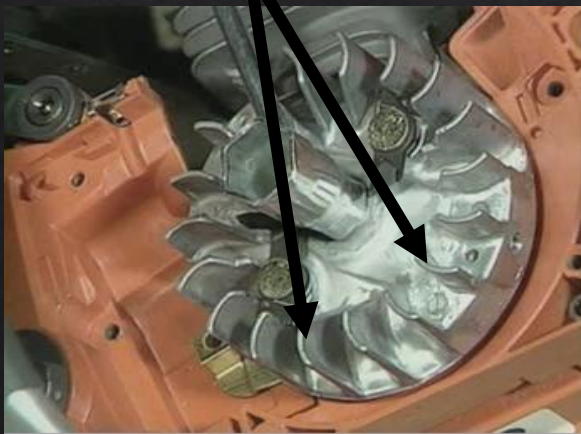
Łopatki wentylatora
