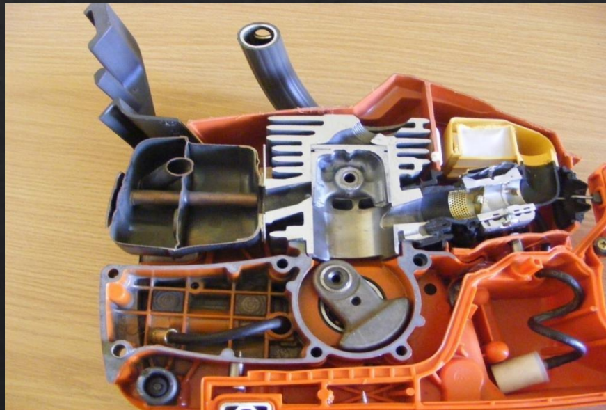
Przekrój silnika spalinowego dwusuwowego pilarki do drewna
