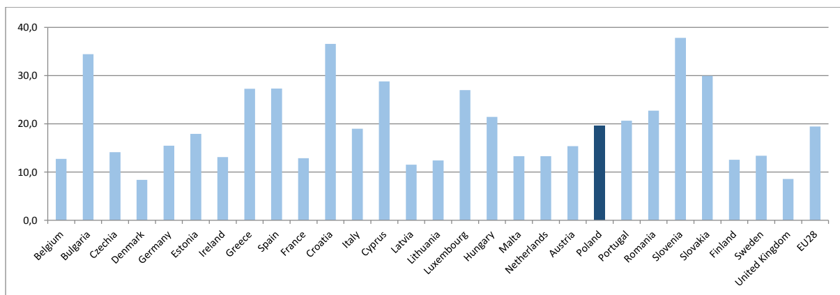
Rys. 8. Udział [%] obszarów Natura 2000 w powierzchni poszczególnych krajów UE
