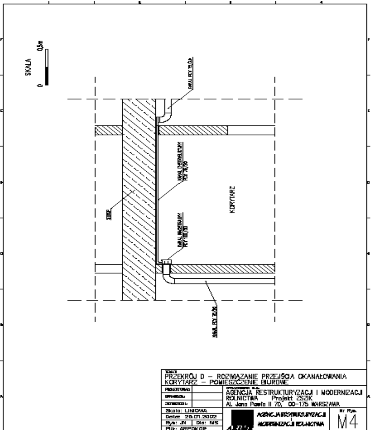
Rysunek 12: Rozwiązanie przejścia okanalowania korytarz-pomieszczenie biurove - nr M4
