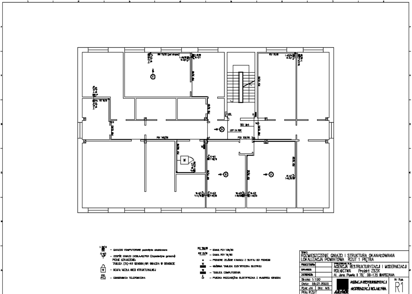
Rysunek 8: Rozmieszczenie gniazd i struktura okanałowania rzut 1-szego piętra - nr R1
