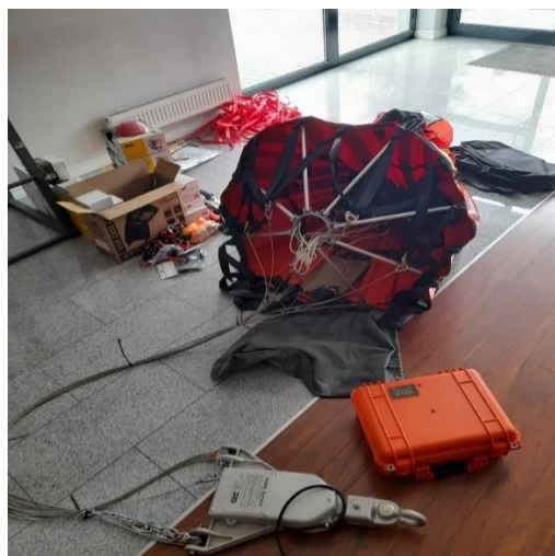
Zdjęcie. Zestaw do gaszenia lasów dla specjalistycznych grup ratownictwa wysokościowego.
