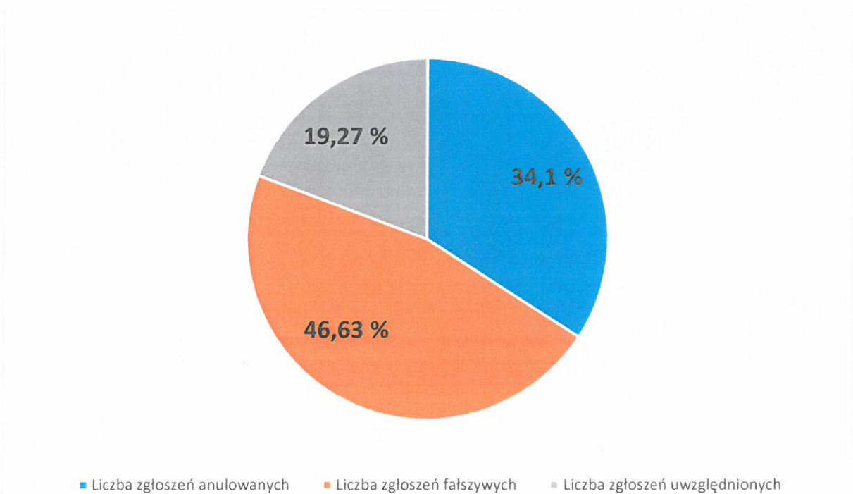
Rysunek 12. Procentowy udział zgłoszeń anulowanych, fałszywych, zasadnych w stosunku do wszystkich połączeń w 2016 r.
