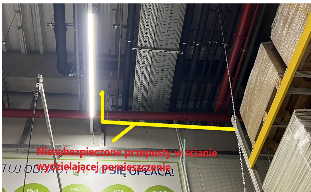
Zdjęcie 1. Brak zabezpieczenia przepustów instalacyjnych w ścianie oddzielenia przeciwpożarowego.
