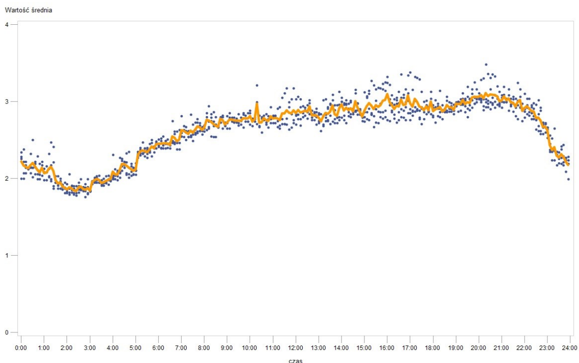
Rys. 6 Wyniki pomiarów – Szkoła Podstawowa nr 8 w Siemianowicach Śląskich – średnia za okres 24 godzin
