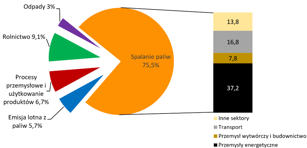
Rys. 3.6. Udział poszczególnych kategorii źródeł w całkowitej emisji krajowej gazów cieplarnianych w 2020 r. Źródło: IOŚ-PIB/KOBiZE
