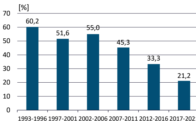
Rys. 8.9. Procent obiektów przemysłowych przekraczających poziomy dopuszczalne – trendy Źródło: GIOŚ/PMŚ
