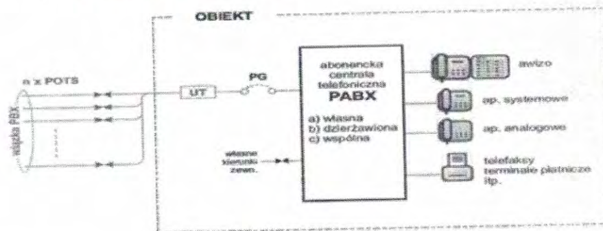
Dostęp POTS/PSTN z wiązkami PBX
