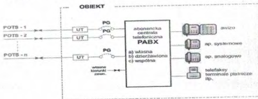
Indywidualne łącza POTS/PSTN
