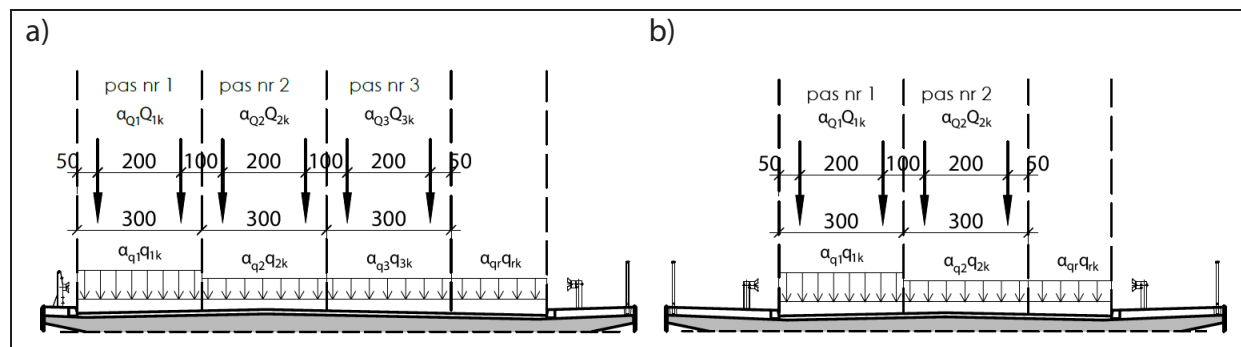
Rys. Z4-2. Schemat ustawienia obciążenia ruchomego LM1: a) na jezdniach dróg klasy A, S, b) na jezdniach dróg klasy G, GP, Z, L, D
