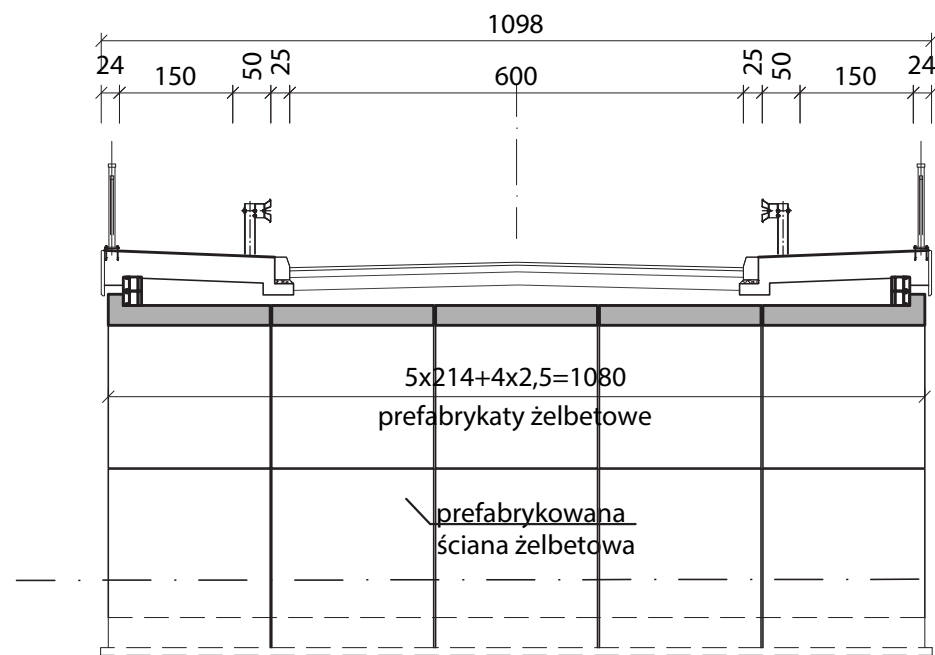
Przekrój poprzeczny dla drogi klasy D - schemat
