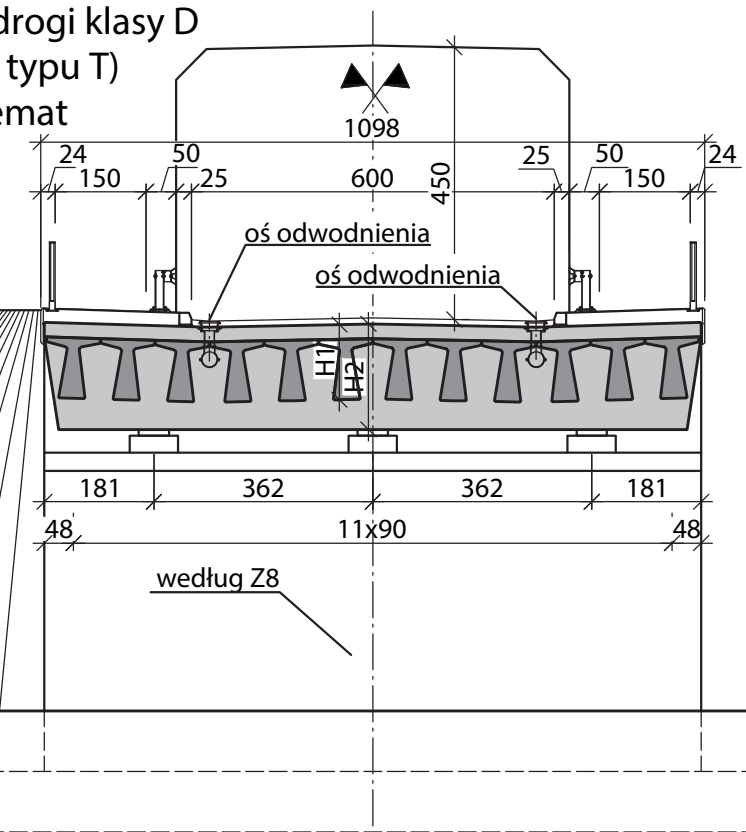
Przekrój poprzeczny obiektu w ciągu drogi klasy D (belki typu ⊥) - schemat
