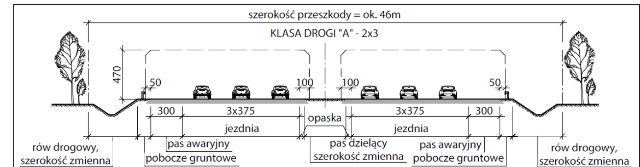
Rys. 3-2. Droga klasy „A” o przekroju 2 x 3
