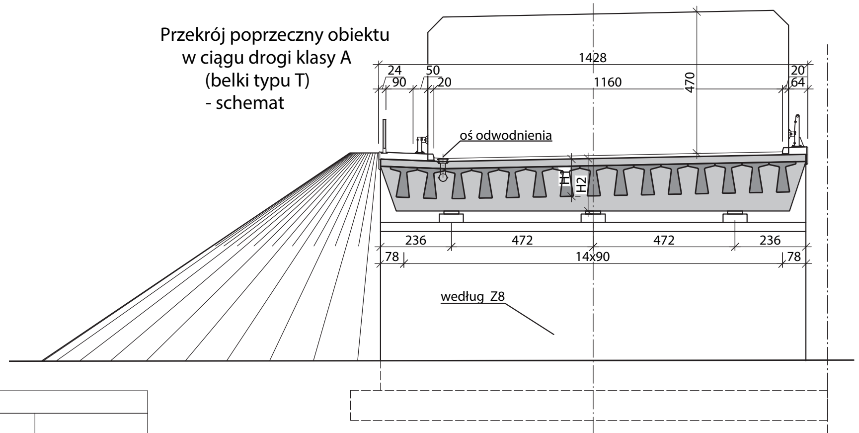
Przekrój poprzeczny obiektu w ciągu drogi klasy A (belki typu ⊥) - schemat
