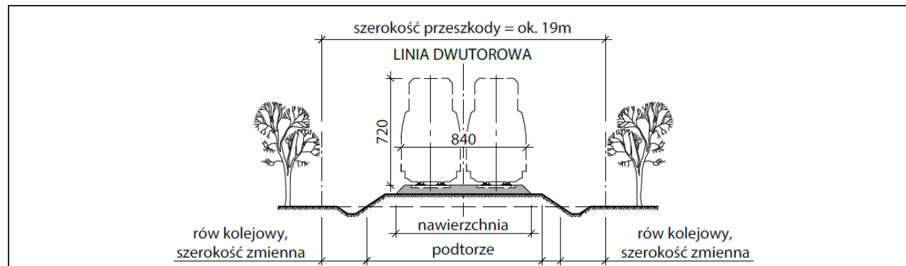
Rys. 3-14. Linia magistralna dwutorowa
