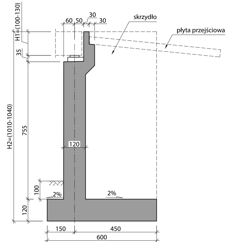
Przekrój poprzeczny
