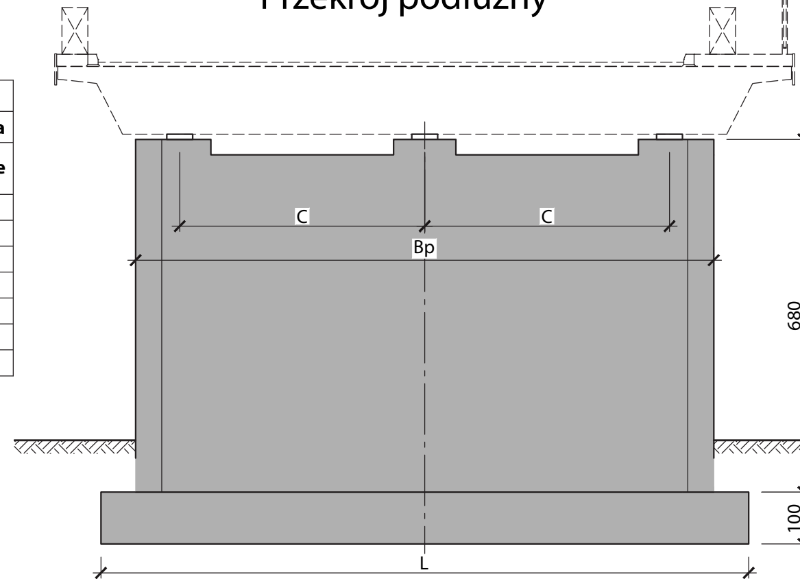
Przekrój podłużny
