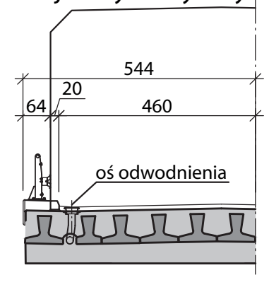
Przekrój niesymetryczny
