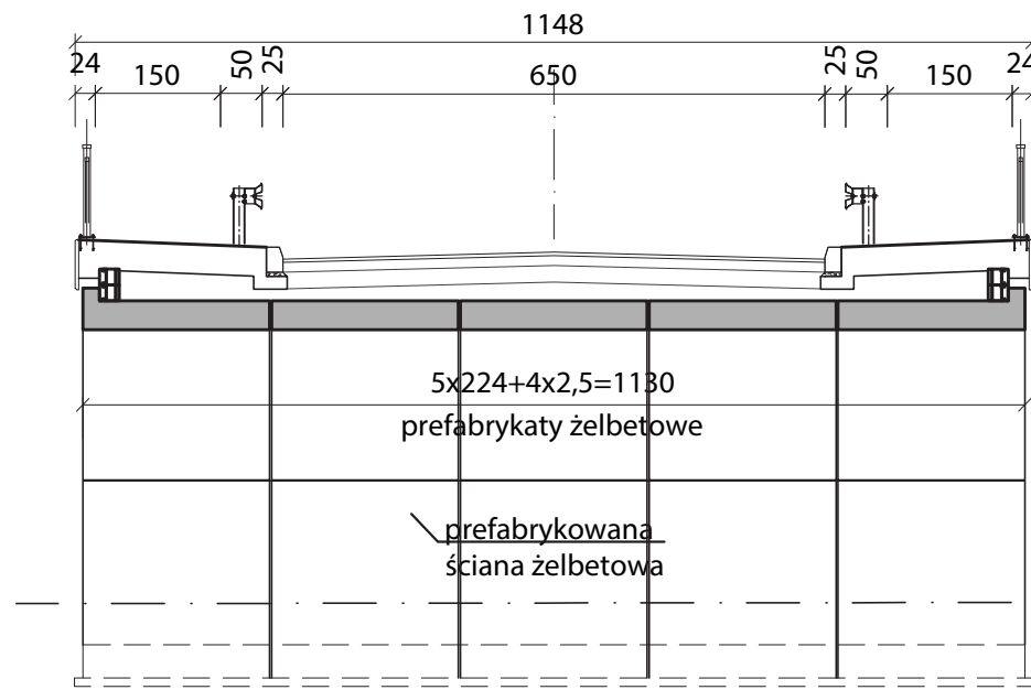
Przekrój poprzeczny dla drogi klasy D - schemat
