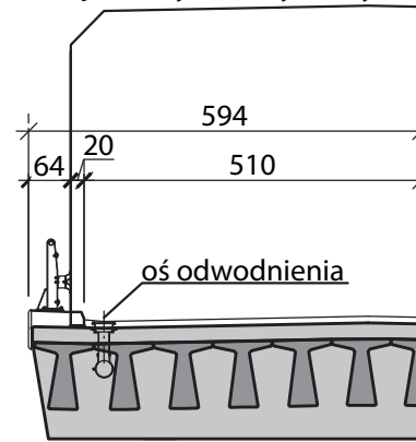
Przekrój niesymetryczny
