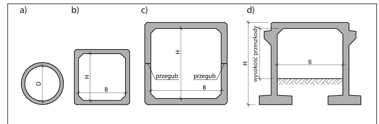
Rys. Z1-2. Schemat konstrukcji: a) przepust kołowy, b) przepust kwadratowy, c) przepust dwuczęściowy, d) mały most
