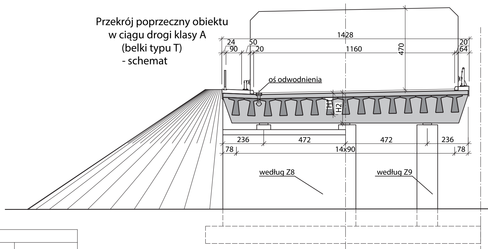
Przekrój poprzeczny obiektu w ciągu drogi klasy A (belki typu L) - schemat
