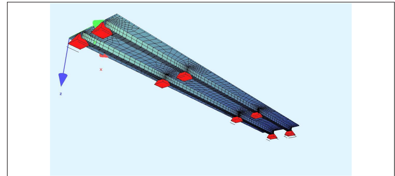
Rys. Z7-2. Wizualizacja modelu obliczeniowego – obiekt trzyprzęsłowy
