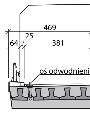
Przekrój niesymetryczny
