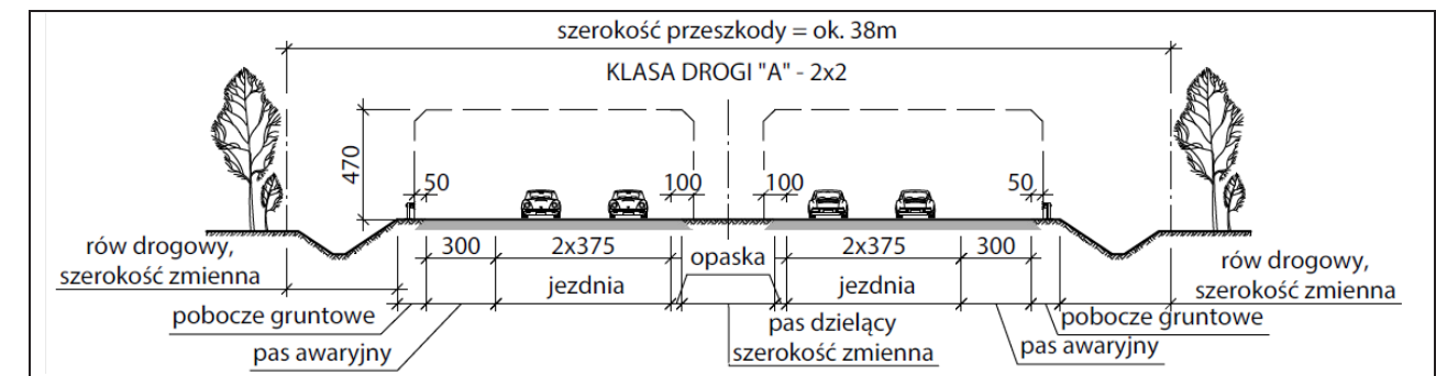
Rys. 3-1. Droga klasy „A” o przekroju 2 x 2
