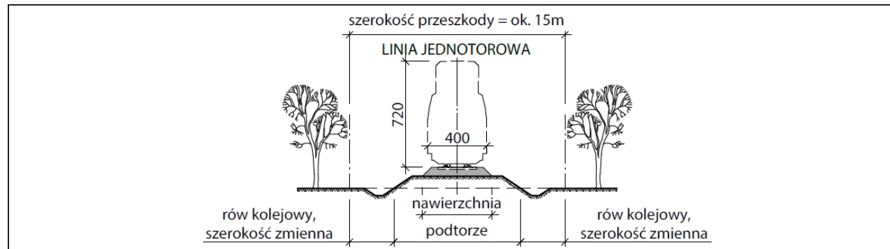
Rys. 3-13. Linia magistralna jednotorowa
