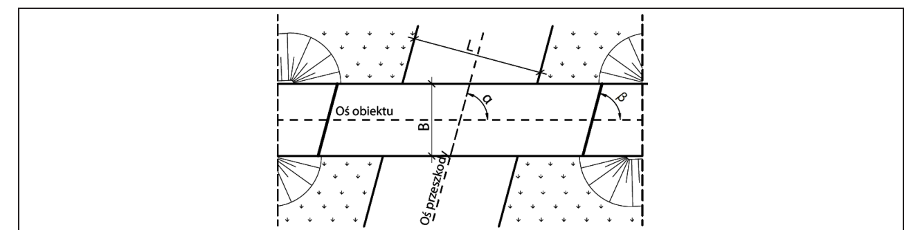
Rys. 3-17. Sposób określania kąta skosu obiektu \beta
