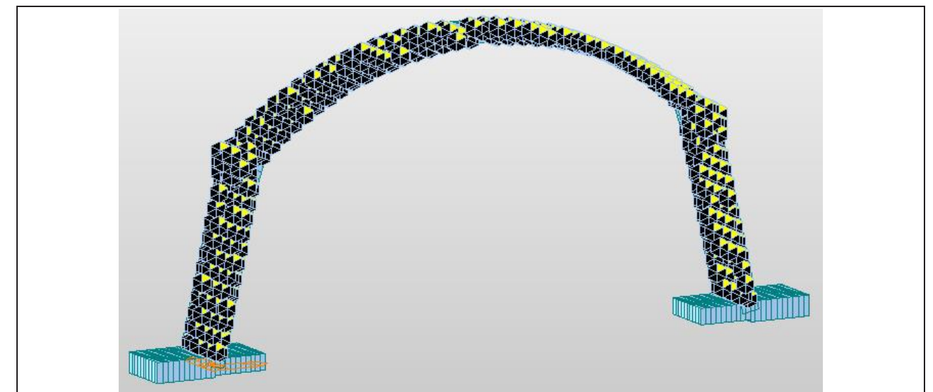
Rys. Z2-3. Wizualizacja modelu obliczeniowego obiektu
