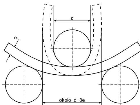
Schemat próby zginania
