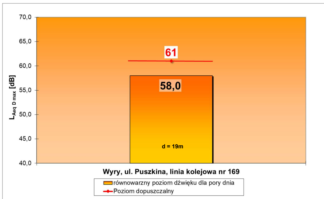
Ryc. 2. Wartość wskaźnika L_{Aeq,D} dla rozpatrywanego punktu referencyjnego oraz jego porównanie z obowiązującą wartością poziomu dopuszczalnego, Wyry, 2022 rok.
