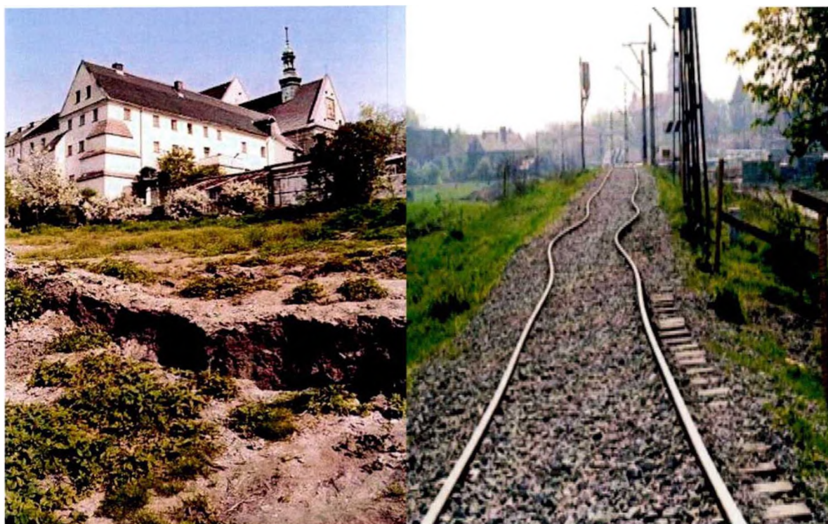
Rys.10i 11Szkody na powierzchni w niecce osiadań w rejonie Klasztoru o.o. Franciszkanów-Reformatów i linii kolejowej
