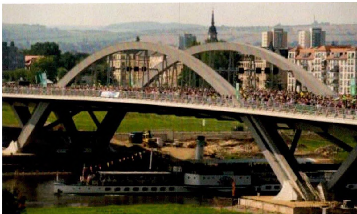
Rys. 3 Most na łacie w Dreźnie
