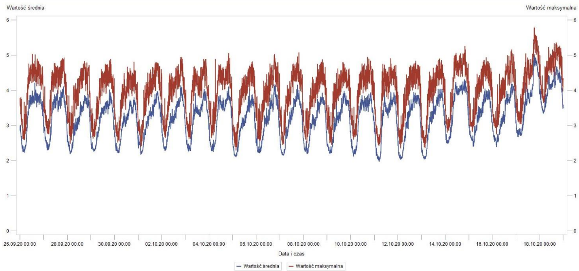
Rys. 5 Wyniki pomiarów – SP nr 20 w Gorzowie Wielkopolskim w okresie 26.09.2020 r. – 18.10.2020 r.
