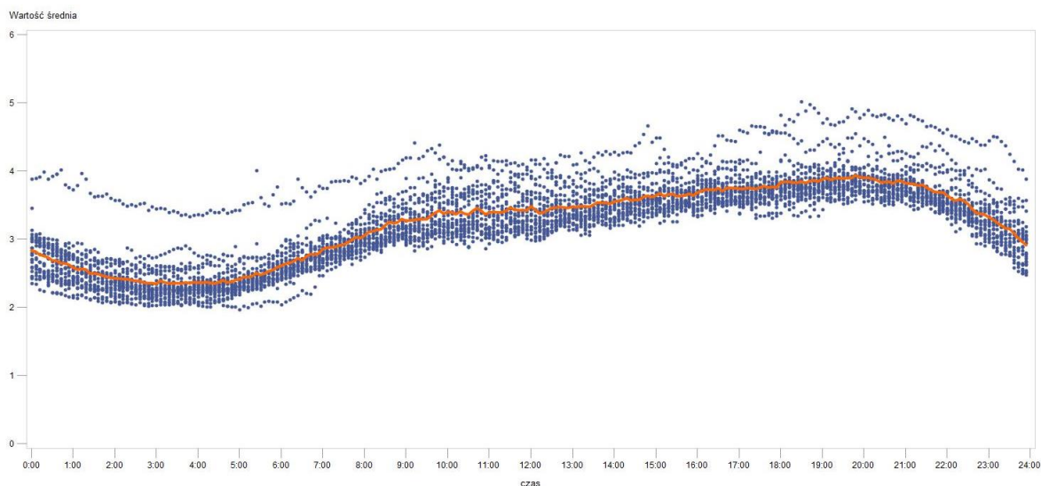
Rys. 7 Wyniki pomiarów – SP nr 20 w Gorzowie Wielkopolskim – średnia za okres 24 godzin
