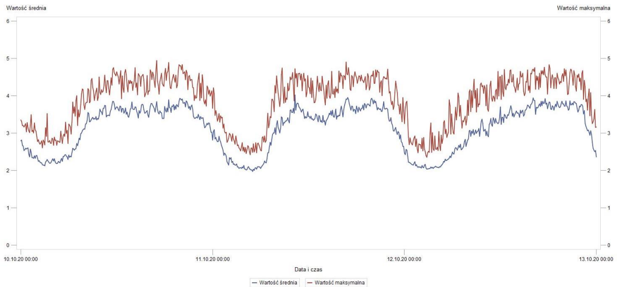
Rys. 6 Wyniki pomiarów – SP nr 20 w Gorzowie Wielkopolskim w okresie 10.10.2020 r. – 12.10.2020 r.
