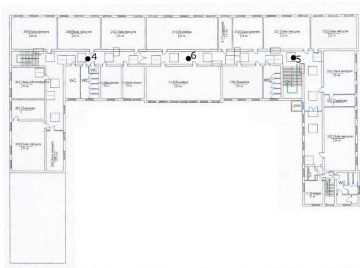
Rys. 1b: Plan rozmieszczenia punktów pomiarowych – 1 piętro
