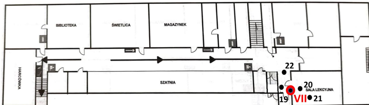
Rys. 1a: Plan rozmieszczenia punktów pomiarowych – Piwnica kolorem czerwonym oznaczono lokalizację punktów dostępnych
