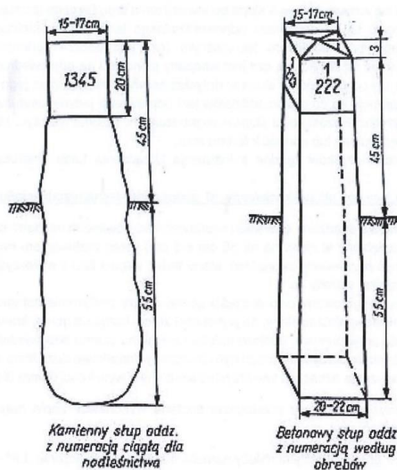
Rysunek 1. Parametry słupa kamiennego i betonowego wraz z oznaczeniem słupa oddziałowego.
