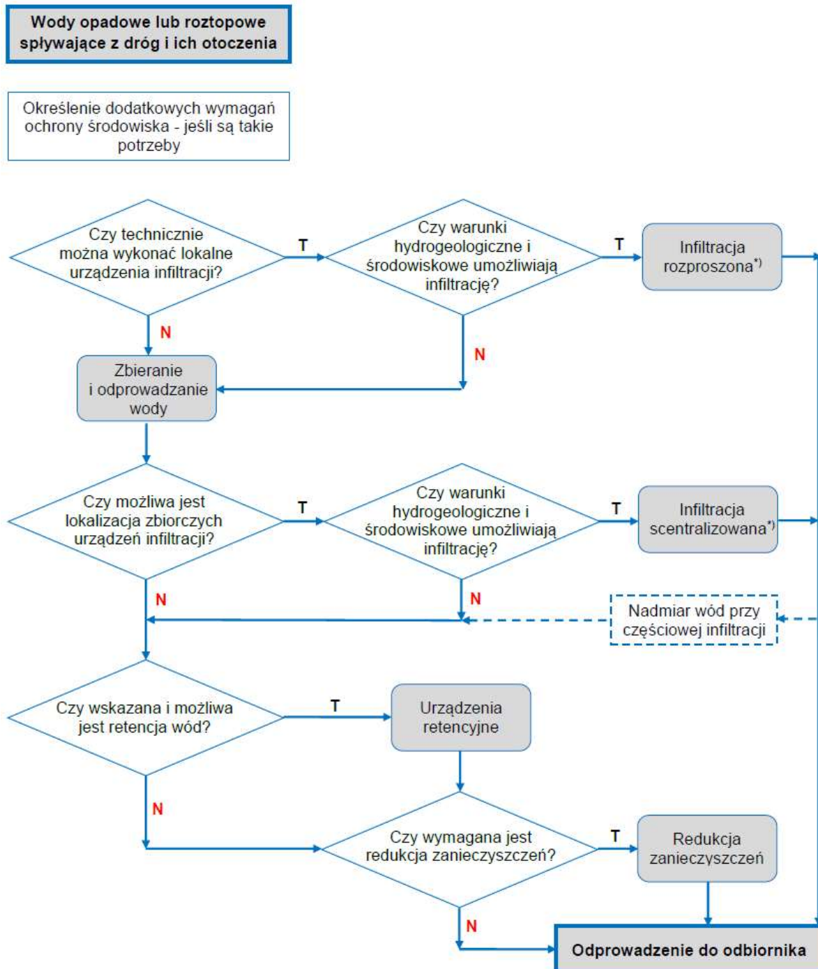
Rys. 4.1.3. Schemat blokowy wyboru sposobu odprowadzenia wód opadowych lub roztopowych (opracowanie własne na podstawie [11])
