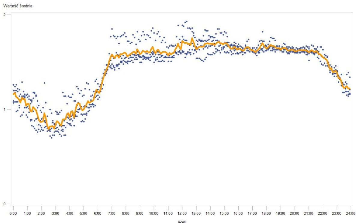
Rys. 7 Wyniki pomiarów – Zespół Szkół w Suwałkach – średnia za okres 24 godzin
