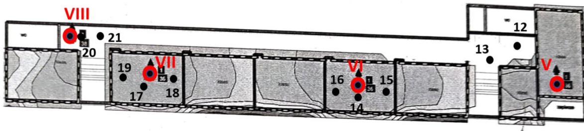
Rys. 1b: Plan rozmieszczenia punktów pomiarowych – I Piętro kolorem czerwonym oznaczono lokalizację punktów dostępnych
