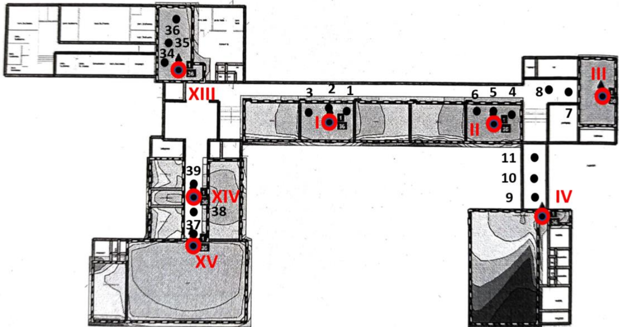
Rys. 1a: Plan rozmieszczenia punktów pomiarowych – Parter kolorem czerwonym oznaczono lokalizację punktów dostępnych
