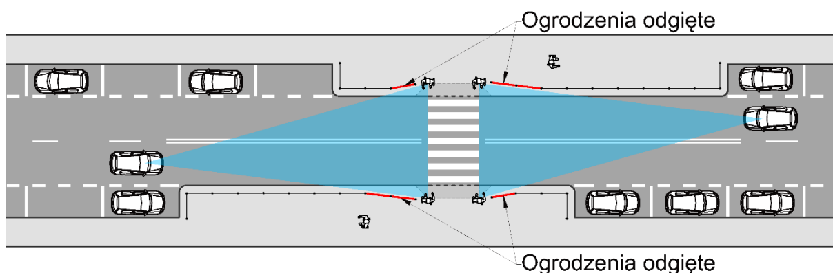
Rys. 14.7.1. Zapewnienie pól widoczności poprzez odgięcie ogrodzeń
