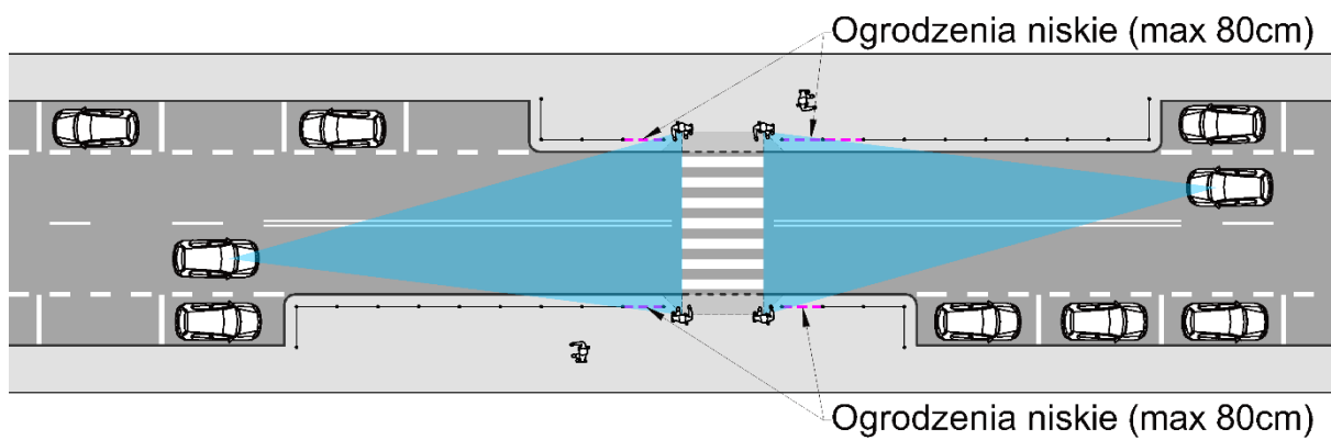
Rys. 14.7.2. Zapewnienie pól widoczności poprzez zastosowanie ogrodzeń niskich
