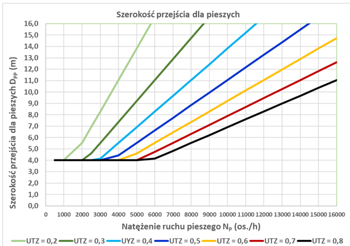
Rys. 10.2.1. Szerokości przejść dla pieszych z sygnalizacją świetlną D_{pp} w zależności od natężenia ruchu pieszego N_p i udziału światła zielonego dla pieszych w cyklu U_{TZ}
