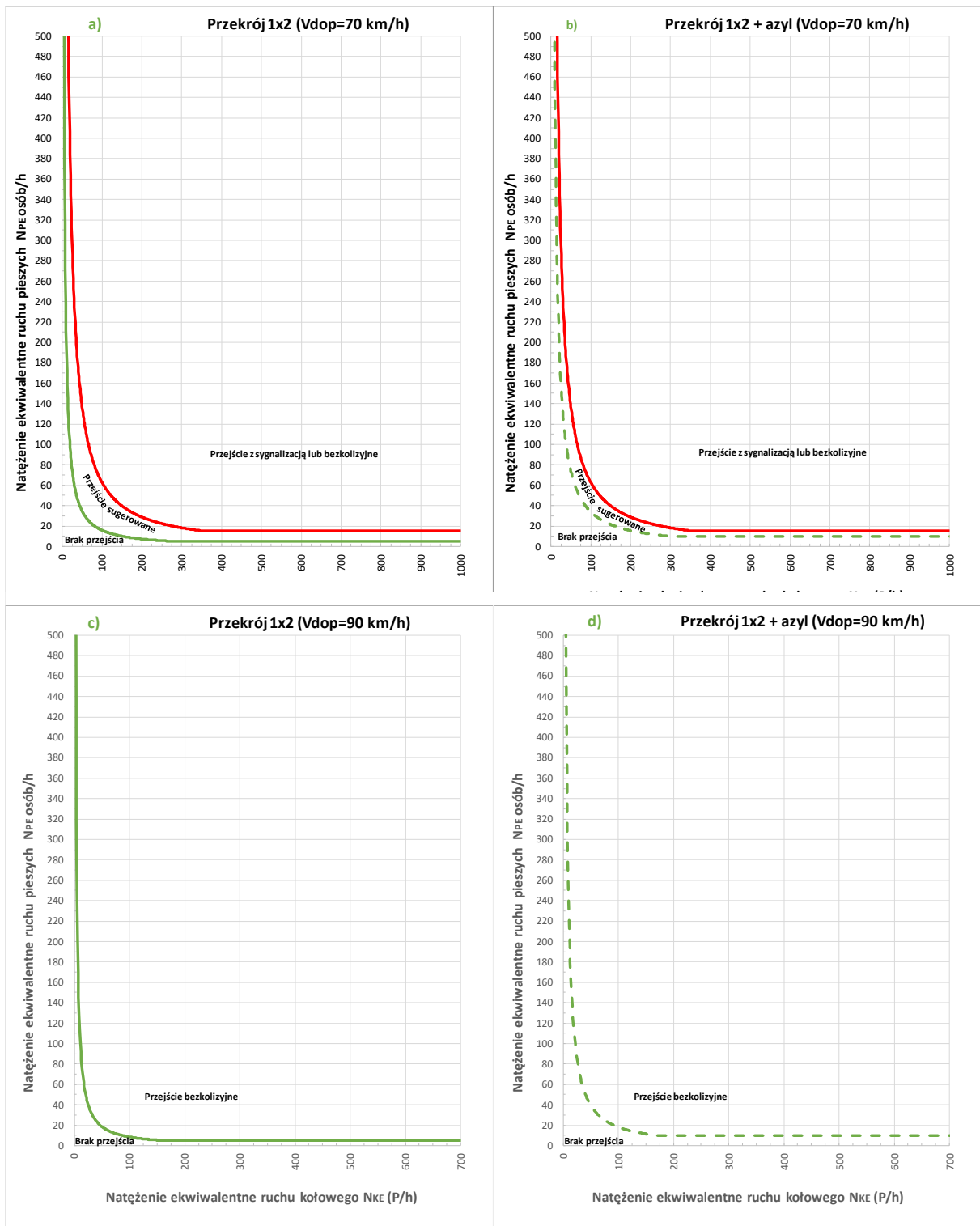
Rys. 8.4.2. Nomogram wyboru rodzaju infrastruktury punktowej dla pieszych przekraczających drogę o: a) V_{dop} = 70 km/h bez wyspy azylu, b) V_{dop} = 70 km/h z wyspą azylu, c) V_{dop} = 90 km/h bez wyspy azylu, d) V_{dop} = 90 km/h z wyspą azylu
