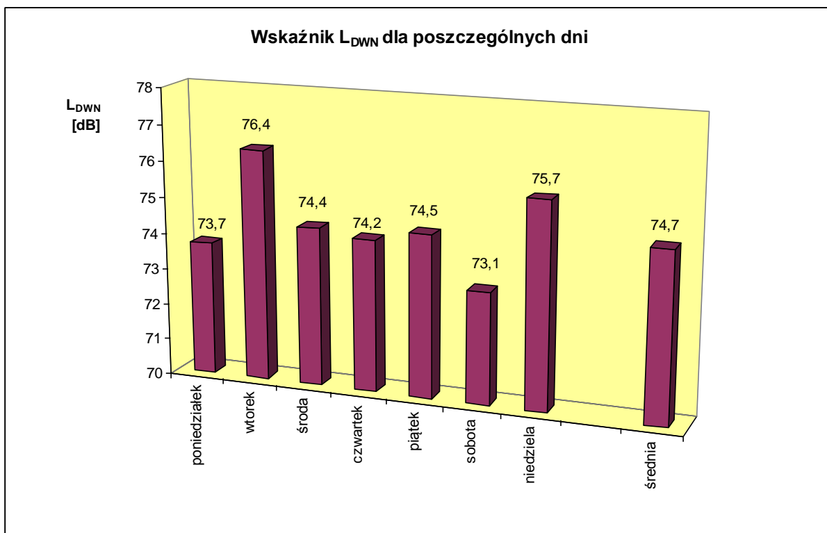
Ryc. 3. Wskaźnik L_{DWN}^{1d} (24 h) w [dB]. Zestawienie zmian średniego wskaźnika poziomu hałasu ( L_{DWN} ) dla danej doby tygodnia w badanym punkcie, Kończyce Małe 2013 r.
