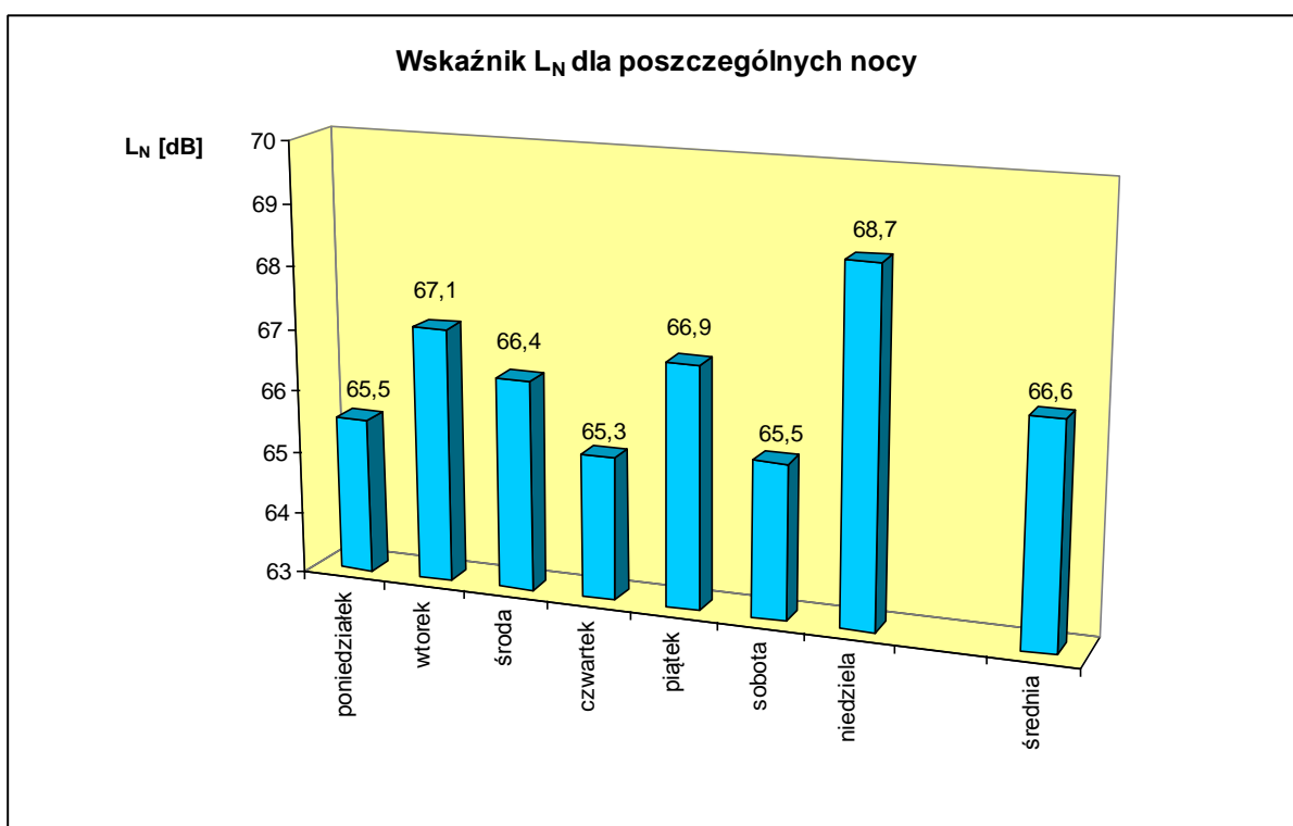
Ryc. 4. Wskaźnik L_N^{1n} (8 h) w [dB]. Zestawienie zmian średniego wskaźnika poziomu hałasu ( L_N ) dla danej nocy tygodnia w badanym punkcie, Kończyce Małe 2013 r.
