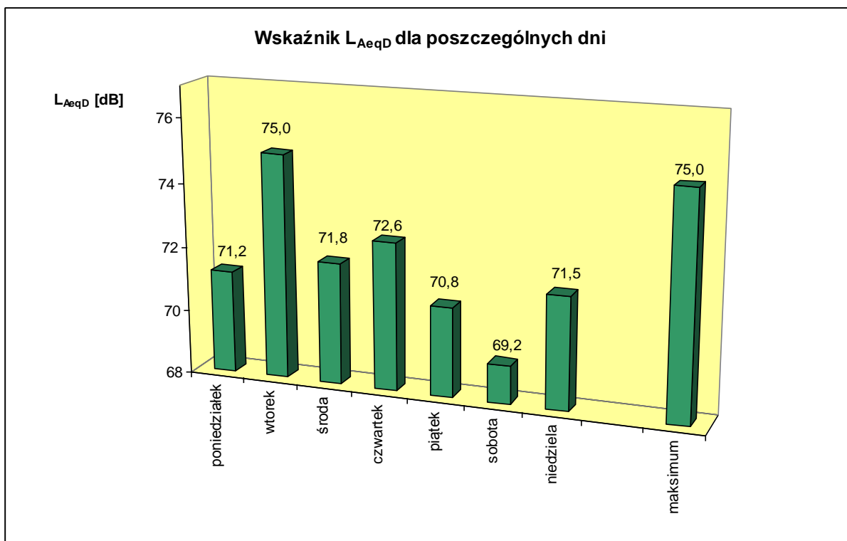
Ryc. 5. Wskaźnik L_{AeqD} (16 h). Zestawienie zmian wskaźnika poziomu hałasu ( L_{AeqD} ), w danym dniu tygodnia oraz jego wartość maksymalna w badanym punkcie, Kończyce Małe 2013 r.
