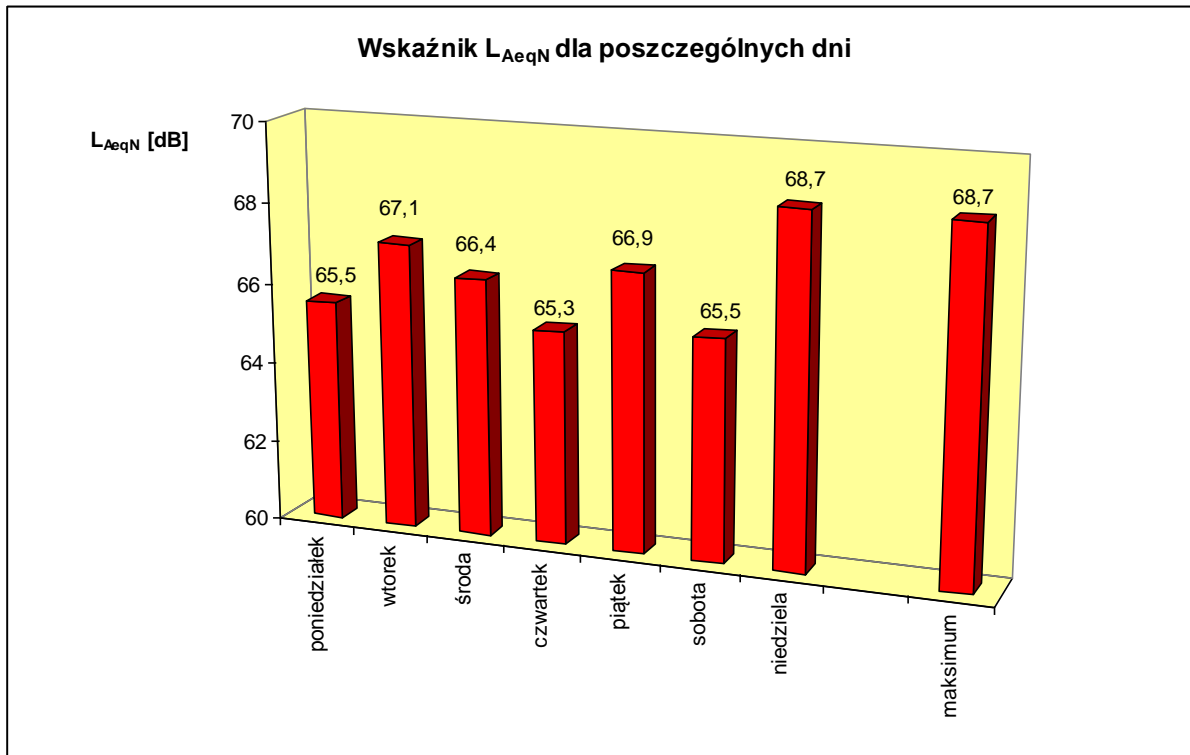
Ryc. 6. Wskaźnik L_{AeqN} (8 h). Zestawienie zmian wskaźnika poziomu hałasu ( L_{AeqN} ), w danym dniu tygodnia oraz jego wartość maksymalna w badanym punkcie, Kończyce Małe 2013 r.
