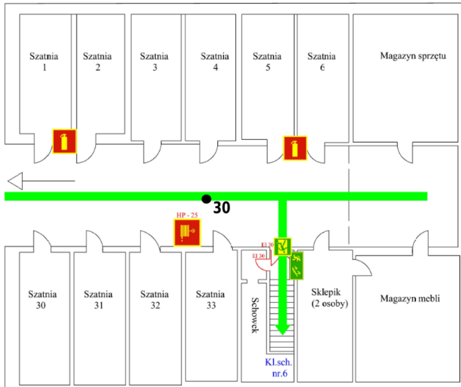
Rys. 1g: Plan rozmieszczenia punktów pomiarowych – piwnica, część D
