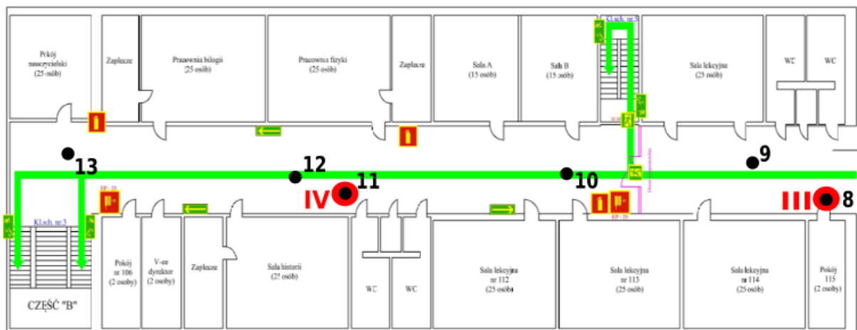
Rys. 1d: Plan rozmieszczenia punktów pomiarowych – I piętro, część E, kolorem czerwonym oznaczono lokalizacje punktów dostępnych
