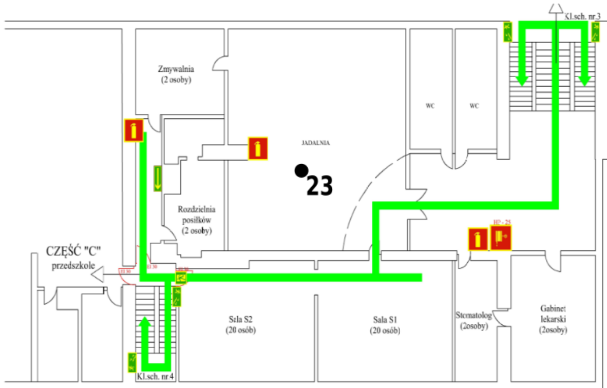
Rys. 1c: Plan rozmieszczenia punktów pomiarowych – I piętro, część B
