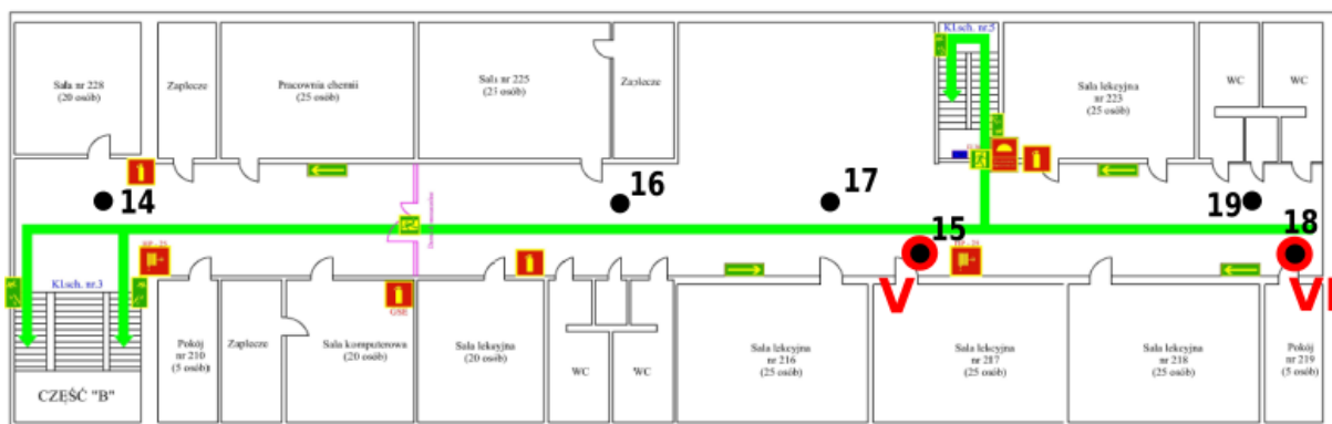
Rys. 1f: Plan rozmieszczenia punktów pomiarowych – II piętro, część E, kolorem czerwonym oznaczono lokalizacje punktów dostępowych
