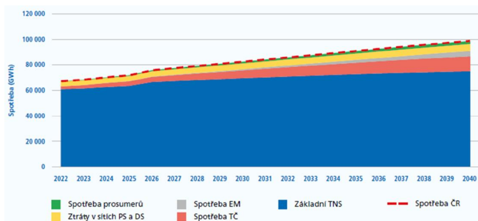
Obr. B.6: Rozwój zużycia energii elektrycznej w RCz - scenariusz progresywny
