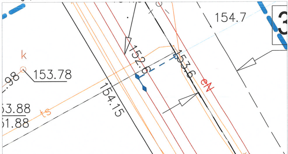
Szczegół, SKALA 1:200
