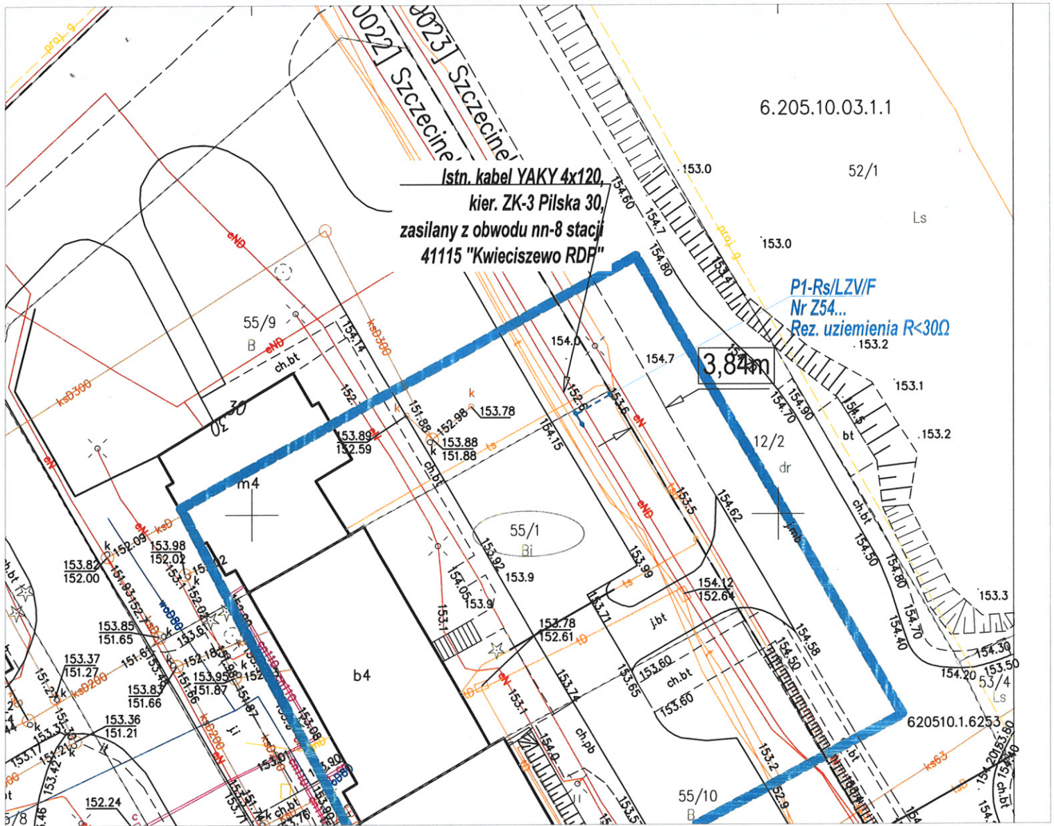
Szczegół, SKALA 1:200
