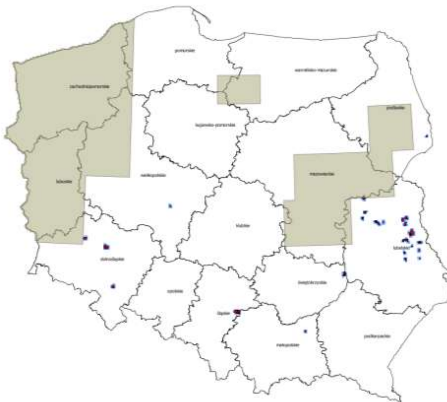
Mapa 4. Obszar aktualizacji ortofotomapy w 2014 r. na podstawie zdjęć lotniczych
