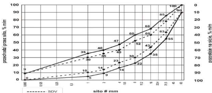
Rys. nr 1. Uziarnienie mieszanki niezwiązanej 0/63 dla podbudowy zasadniczej
