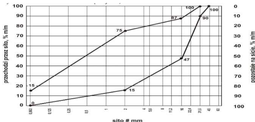
Rys. nr 2. Uziarnienie mieszanki niezwiązanej 0/31,5 dla nawierzchni
