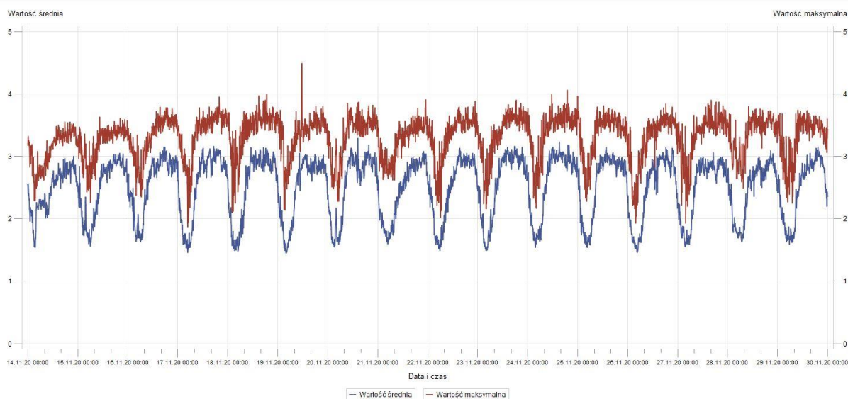
Rys. 5 Wyniki pomiarów – UM Bydgoszcz w okresie 14.11.2020 r. – 29.11.2020 r.
