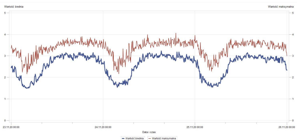
Rys. 6 Wyniki pomiarów – UM Bydgoszcz w okresie 23.11.2020r. – 26.11.2020 r.
