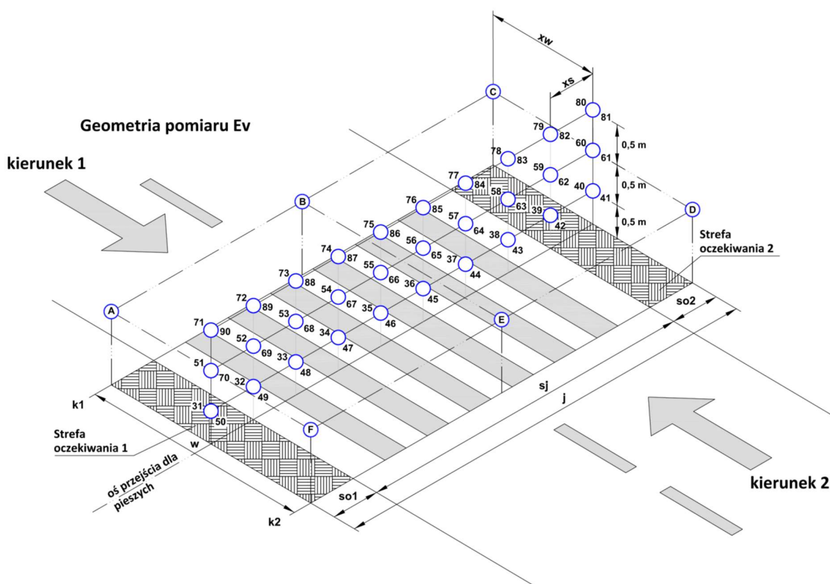
Rys. 6.3.1. Schemat siatki punktów do pomiaru natężenia oświetlenia niezbędnego do określenia klasy oświetleniowej PC (oświetlenie dedykowane) oświetlenia w płaszczyźnie pionowej (E.) na przejściu dla pieszych
