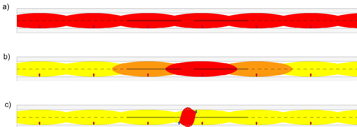
Rys. 3.1.3. Schemat rozmieszczenia opraw oświetlenia w obszarze przejścia dla pieszych: a) rozwiązanie standardowe, b) rozwiązanie standardowe ze strefą przejściową, c) rozwiązanie dedykowane
