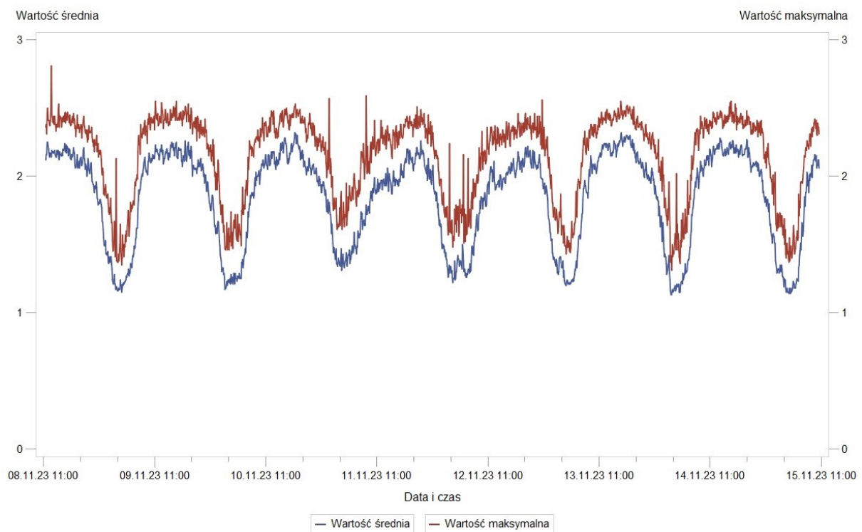
Rys. 5 Wyniki pomiarów – USC w Katowicach w dniach 8.11.2023 r. – 15.11.2023 r. – wartość średnia i wartość maksymalna
