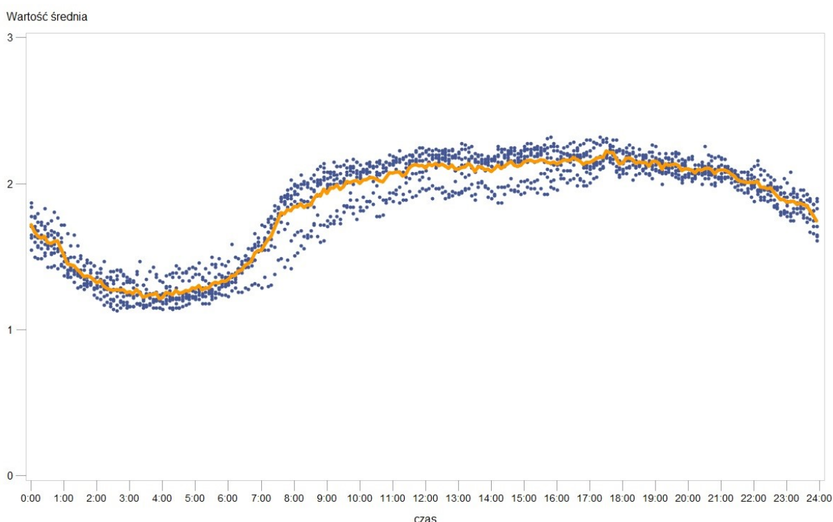
Rys. 6 Wyniki pomiarów – USC w Katowicach – średnia za okres 24 godzin
