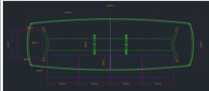
Rys. 1 Rysunek techniczny stołu
