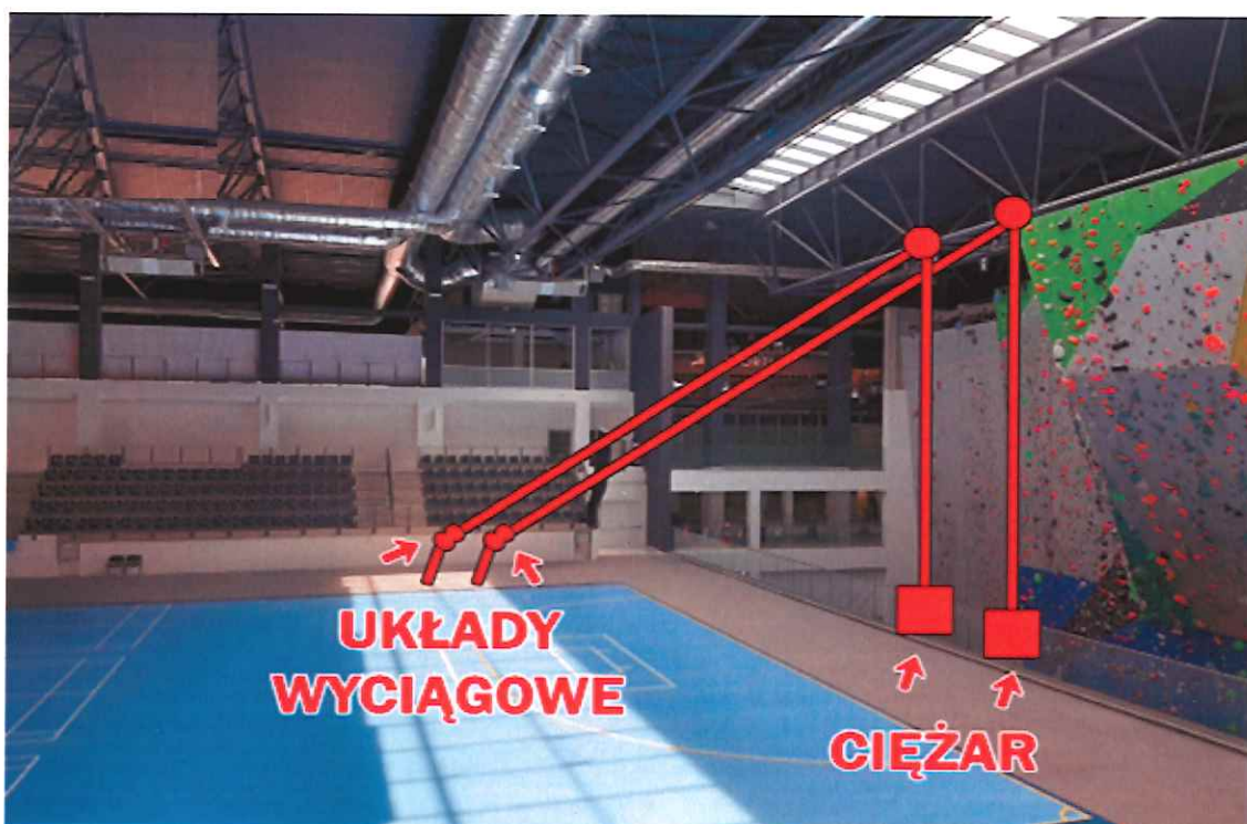
Zdjęcie nr 4: Wielokrążek podstawowy – wyciąganie ciężaru na wysokość około 5 m.
