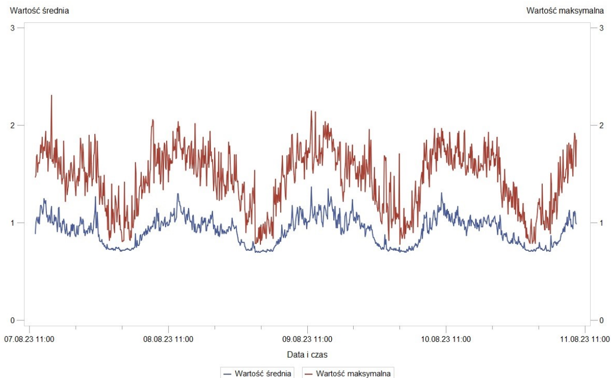
Rys. 6 Wyniki pomiarów – Przedszkole Publiczne nr 13 w Tarnowie w dniach 7.08.2023 r. – 11.08.2023 r. – wartość średnia i wartość maksymalna
