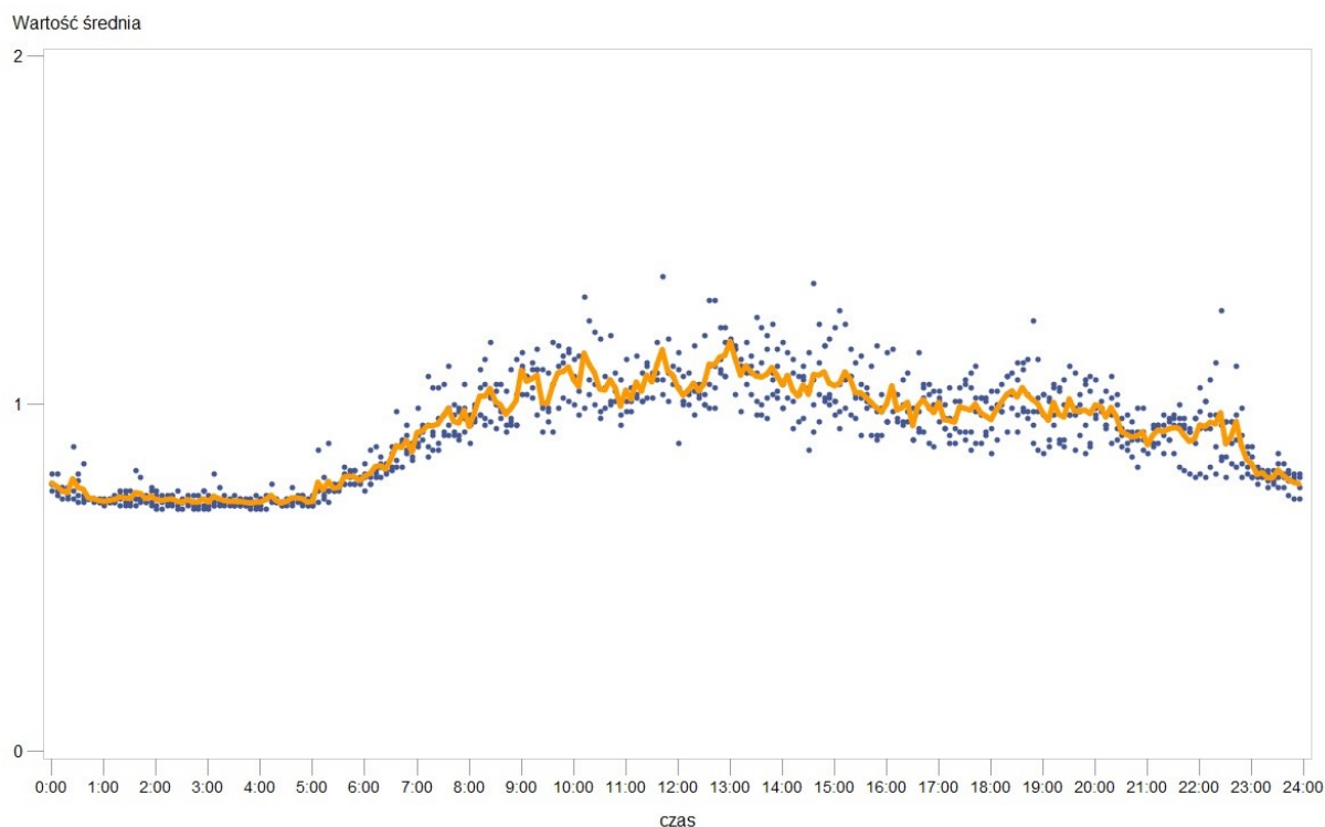
Rys. 7 Wyniki pomiarów – Przedszkole Publiczne nr 13 w Tarnowie – średnia za okres 24 godzin
