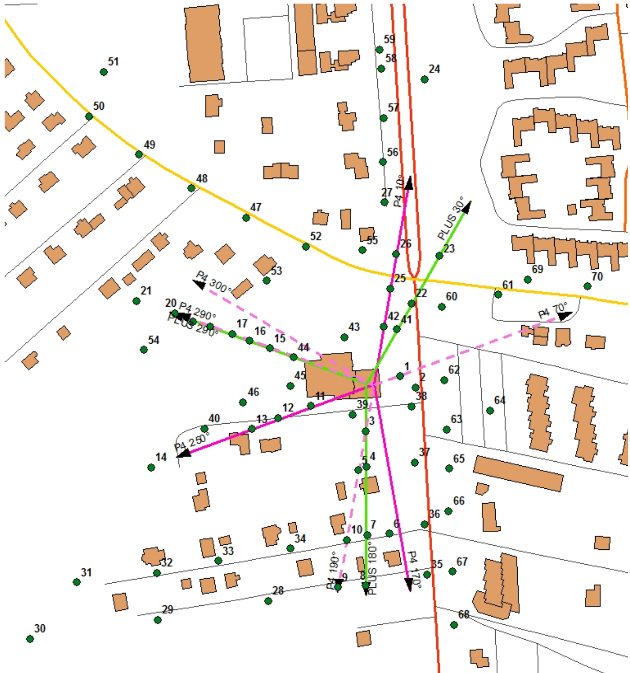
Rys. 1: Plan terenu, na którym znajdują się badane stacje bazowe Uwaga: Linie wyznaczające azymuty anten mają długość 150 m.
