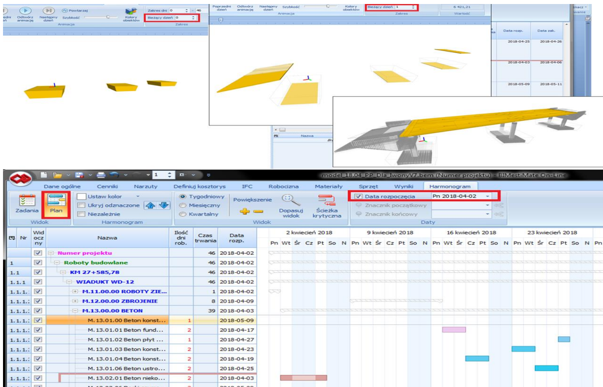
Rys. 5.3.3. Powiązanie harmonogramu z modelem BIM 4D wiaduktu
