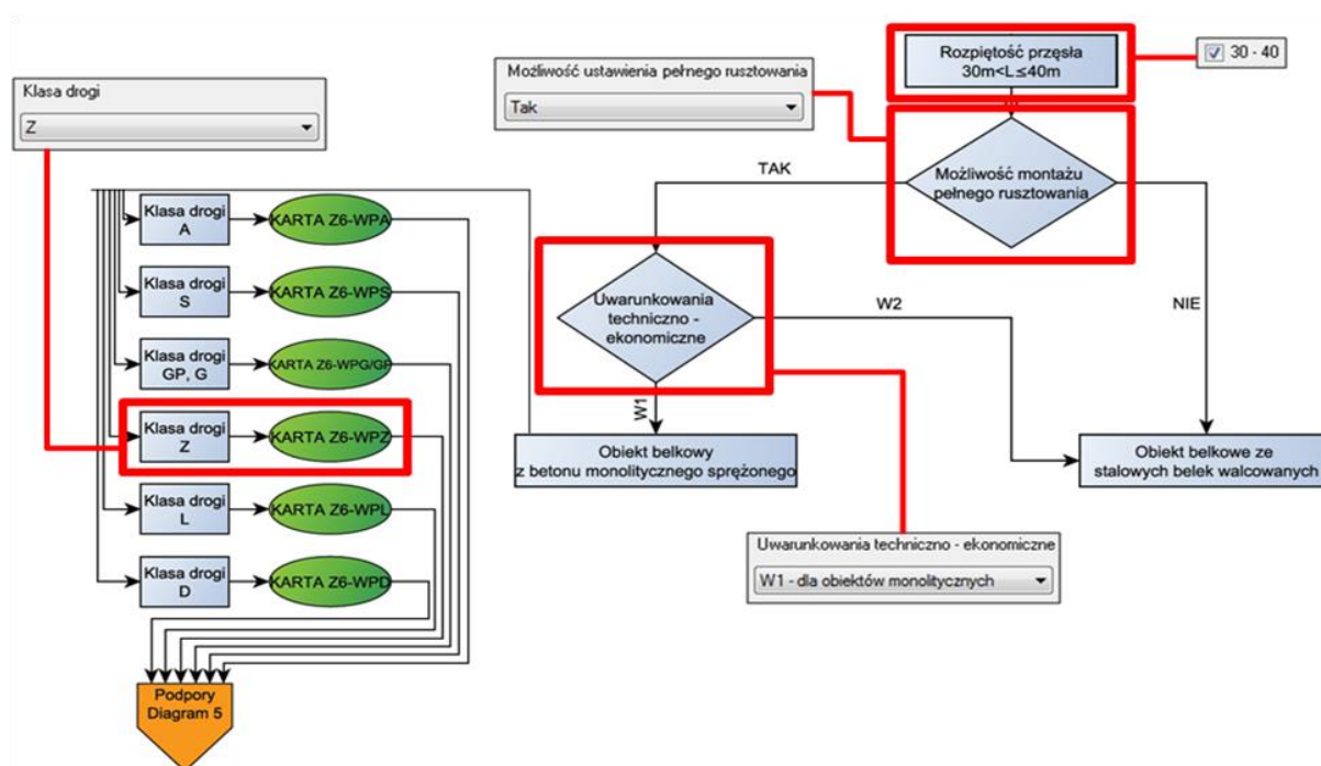
Rys. 5.2.5. Automagiczne generowanie modeli BIM i MES [63] na podstawie WR-M-21-1.
