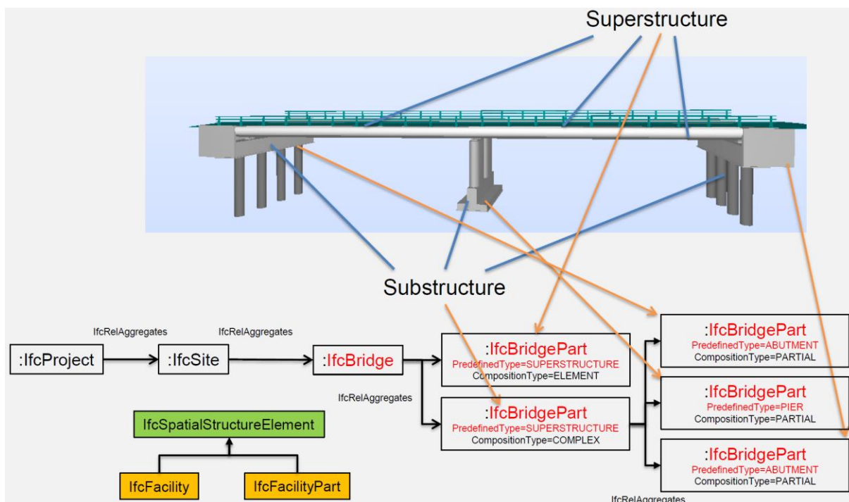
Rys. 7.2.2. Przykład podział modelu mostu na podstawowe komponenty zgodnie z IFC 4 × 2 [51]
