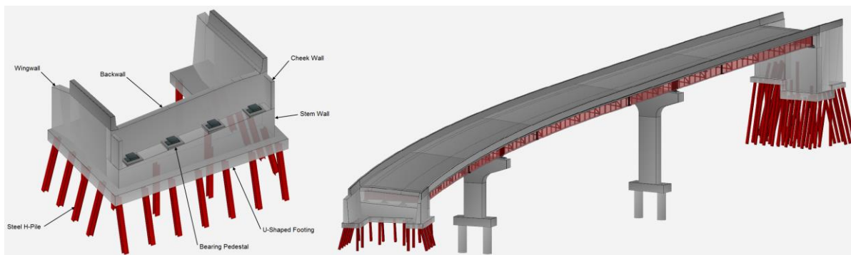
Rys. 7.2.1. Przykład modelowania parametrycznego mostu zgodnie z protokołem openBrIM [35]
