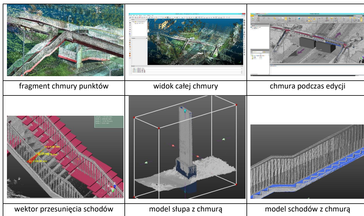
Rys. 5.3.4. Przykład chmury punktów uzyskanej ze skaningu laserowego mostu dla pieszych
