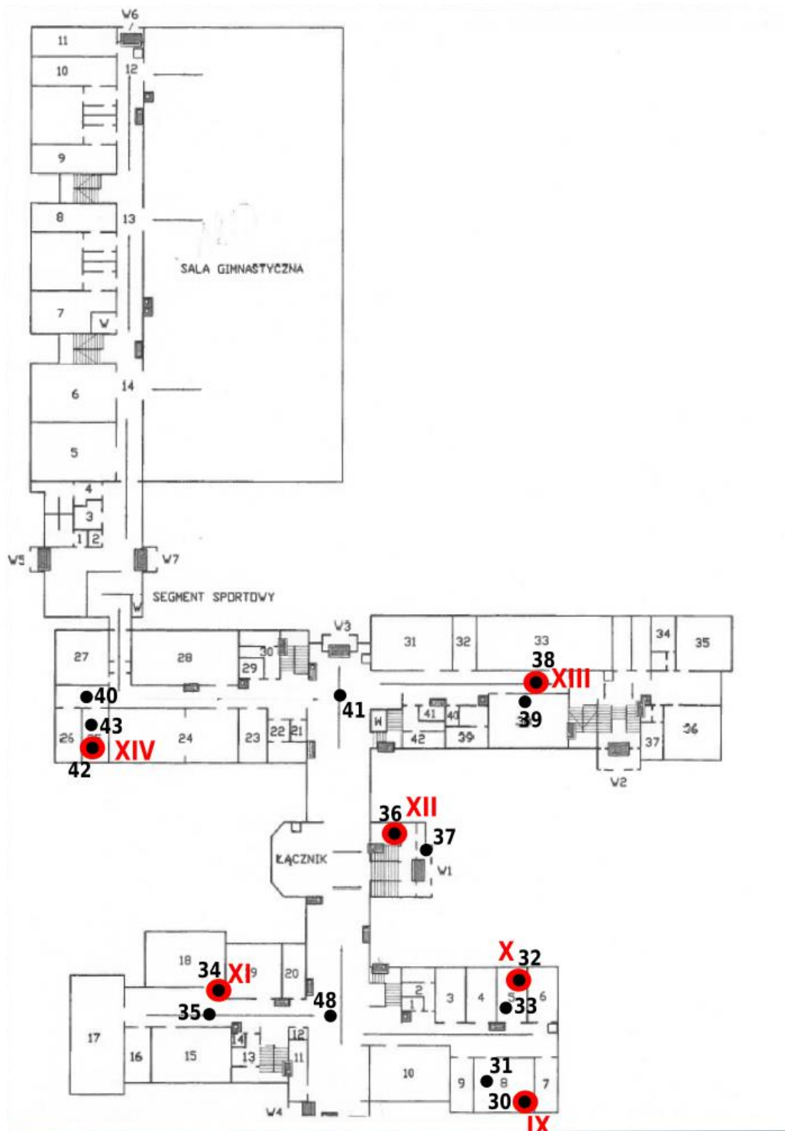
Rys. 1c: Plan rozmieszczenia punktów pomiarowych – parter, kolorem czerwonym oznaczono lokalizacje punktów dostępnych
