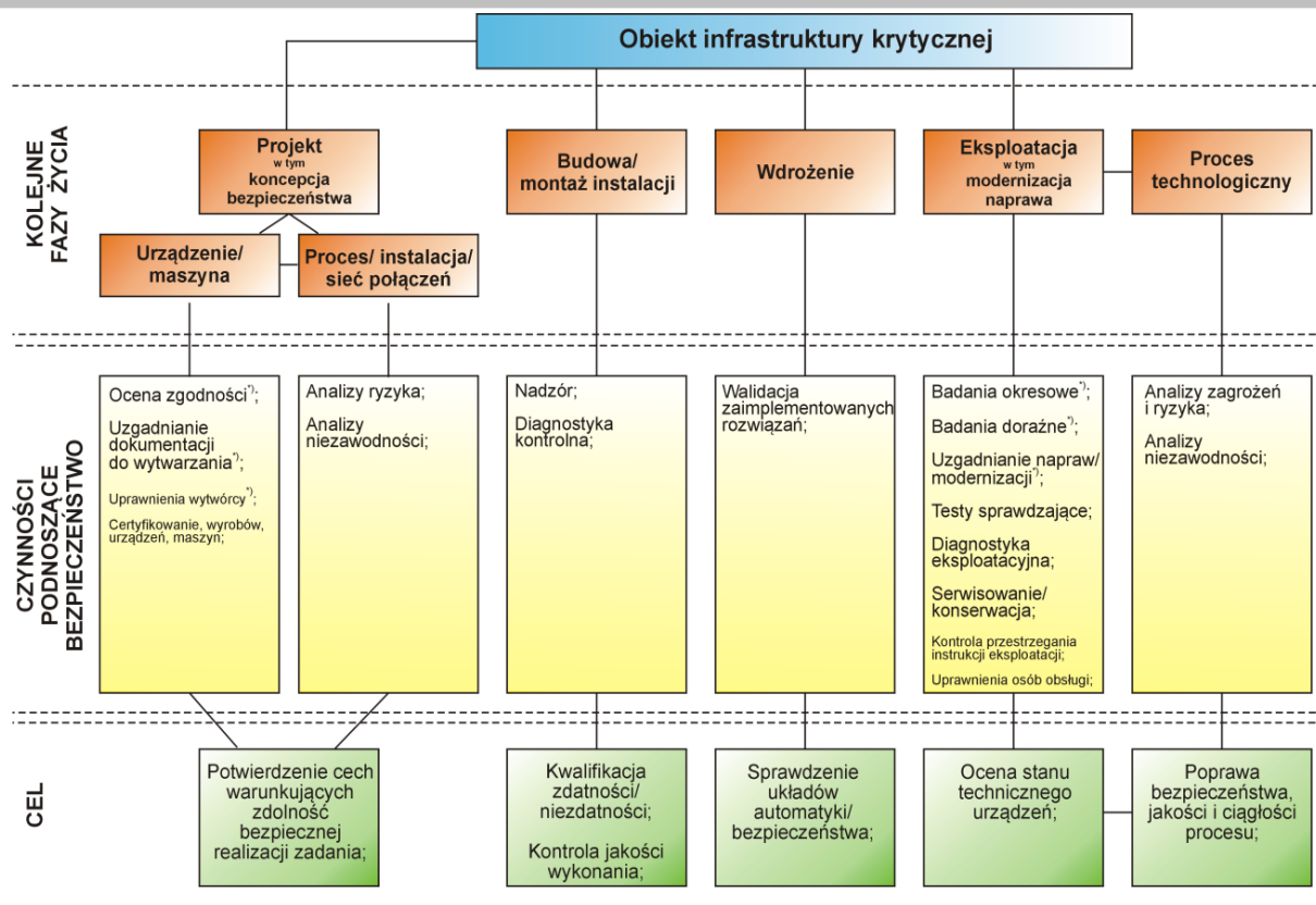
Rys. 10. Wybrane czynności podnoszących bezpieczeństwo obiektów technicznych infrastruktury krytycznej w kolejnych fazach życia 10 .
