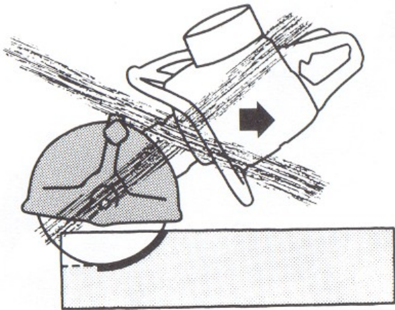
Nieprawidłowy rzaz
