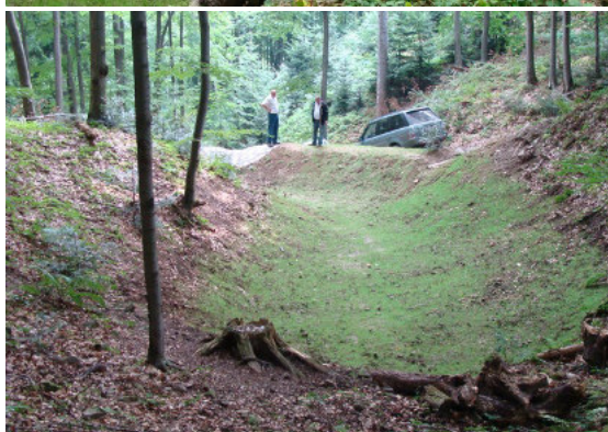
Wspaniałe przykłady wykorzystania naturalnego ukształtowania terenu, które po drobnych modyfikacjach stanowi idealne miejsce na zbiornik retencyjny – Nadleśnictwo Piwniczna. Źródło: Archiwum CKPŚ
