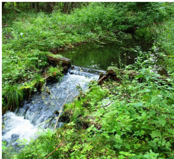
Próg z dwiema ściankami szczelnymi, ubezpieczony palisadą boczną, przelew pomiędzy ściankami, brak ubezpieczenia progu dolnego od strony wody dolnej. Fot. Z. Filipek. Źródło: Archiwum CKPS.
