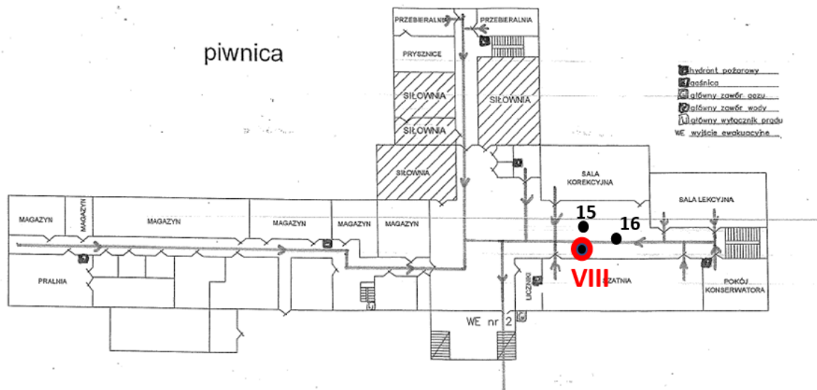
Rys. 1c: Plan rozmieszczenia punktów pomiarowych – piwnica, kolorem czerwonym oznaczono lokalizacje punktów dostępnych
