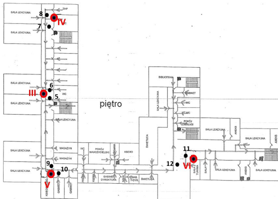
Rys. 1b: Plan rozmieszczenia punktów pomiarowych – I piętro kolorem czerwonym oznaczono lokalizację punktów dostępnych
