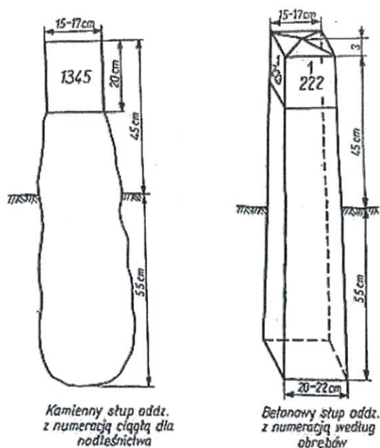
Rysunek 1. Parametry słupka kamiennego i betonowego wraz z oznaczeniem słupa oddziałowego.
