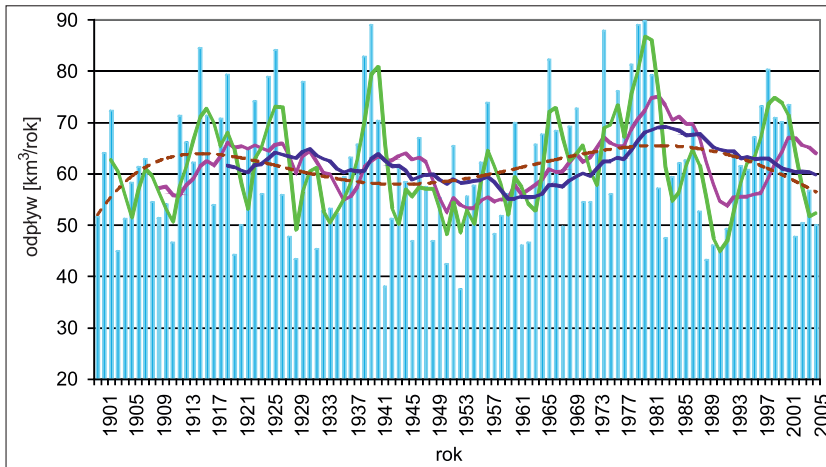
Rys. 5.5-1. Odpływ rzeczny z obszaru kraju w latach 1901-1990 [na podstawie: Fal, 1993 oraz roczników statystycznych GUS]
