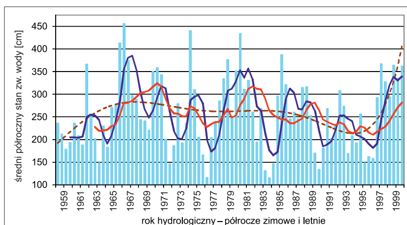
Rys. 5.5-3. Dynamika stanu retencji poziomego w utworach szczelinowo-porowych kredy górnej (kreda pizująca i margle), rejestrowana w posterunku IMGW Anusin k. Chełma w latach 1959-2000 [Herbich, Prażak, Przytuła, 2009a]
