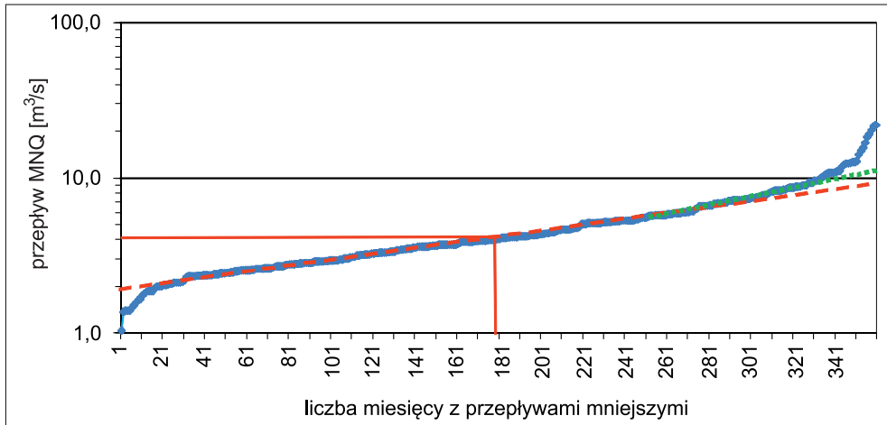
Rys. 5.3-4. Wyznaczenie odpływu podziemnego SQG metodą Killego na krzywej kumulacyjnej zbioru MNQ rzeki Liwiec w Łochowie z wielolecia 1951-1980 jako wartości równej przepływowi MNQ_{(0,5TW)} (gdzie 0,5TW = 180 miesięcy) wraz z mniejszymi: QG = MNQ_{(0,5TW)} = 4,1 \text{ m}^3/\text{s}
