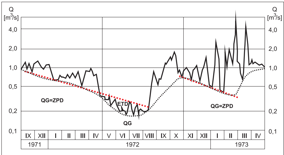
Rys. 5.3-1. Hydrogram przepływu całkowitego rzeki (Wojśławka w Małochwieju) z wydzieleniem zasilania podziemnego doliny rzecznej ( ZPD ) oraz zasilania podziemnego rzeki ( QG ) i drenażu ewapotranspiracyjnego wód podziemnych ( ETD ) w obrębie tarasu niskiego (podmokłego) doliny [Herbich, 1980]
