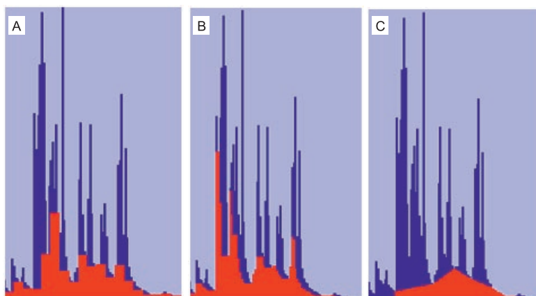
Rys. 5.3-2. Przykłady wydzielenia odpływu podziemnego poprzez podział hydrogramu z uwzględnieniem minimów przepływu występujących w równych przedziałach czasowych (A), okresowych regresji przepływu (B) i lokalnych minimów przepływu (C)
