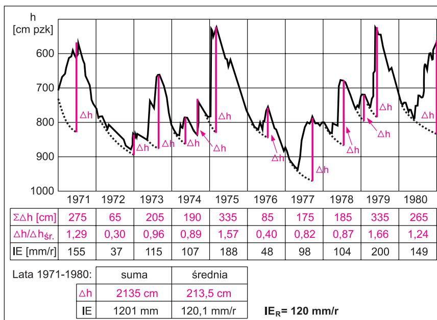
Rys. 5.7-1. Określenie infiltracji efektywnej metodą analizy zmian stanu retencji wód podziemnych
