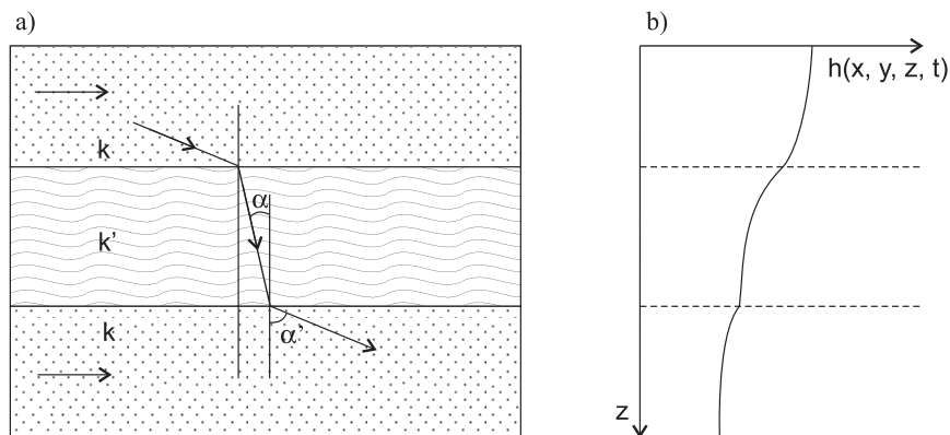
Rys. 6.5-1. Działanie warstwy słabo przepuszczalnej [za: Szymanko, 1980]
