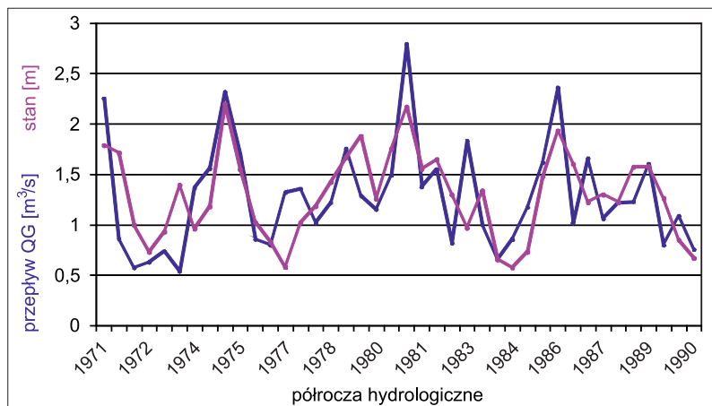
Rys. 5.3-5. Przykład wyraźnego związku stanów retencji i odpływu podziemnego w zlewniach rzek drenujących poziom wodonośny o swobodnym zwierciadle wody
