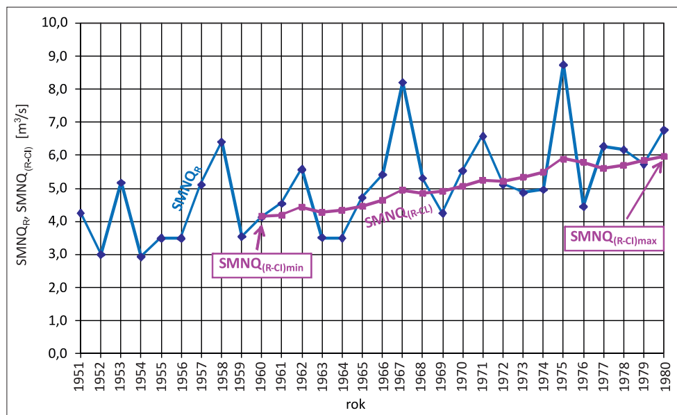
Rys. 5.3-3. Wielkość niskich miesięcznych przepływów Liwca w Łochowie: średnich rocznych SMNQ_R oraz średnich ruchomych SMNQ_{(R-CI)} z okresu poprzedzającego dany rok o czas opóźnienia CI = 10 lat
