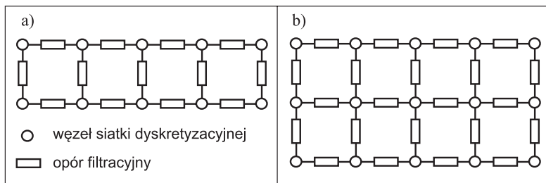
Rys. 6.5-2. Schematy odwzorowania na modelu warstwy słabo przepuszczalnej
