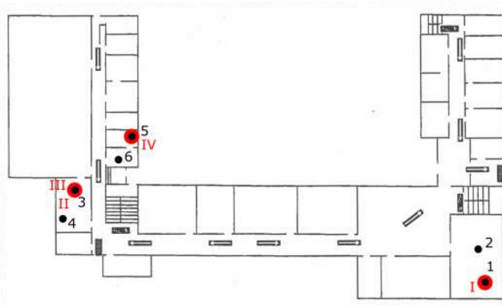
Rys. 1a: Plan rozmieszczenia punktów pomiarowych – parter, część 1, kolorem czerwonym oznaczono lokalizację punktów dostępnych
