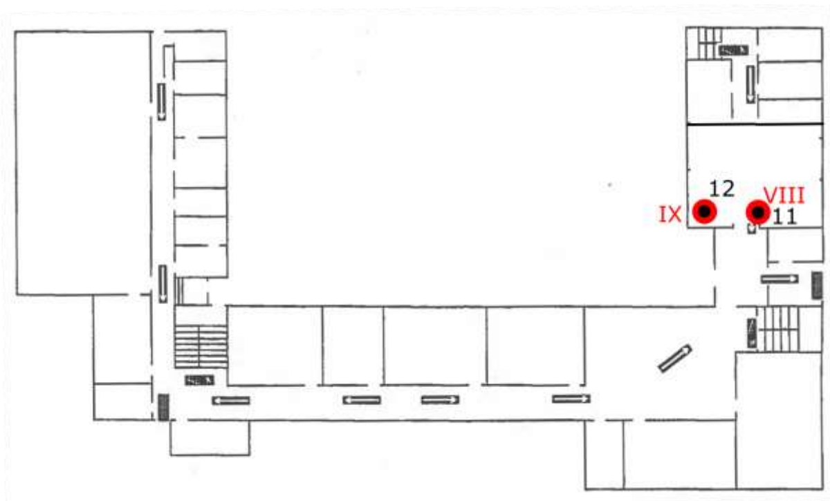
Rys. 1d: Plan rozmieszczenia punktów pomiarowych – II piętro, kolorem czerwonym oznaczono lokalizację punktów dostępnych
