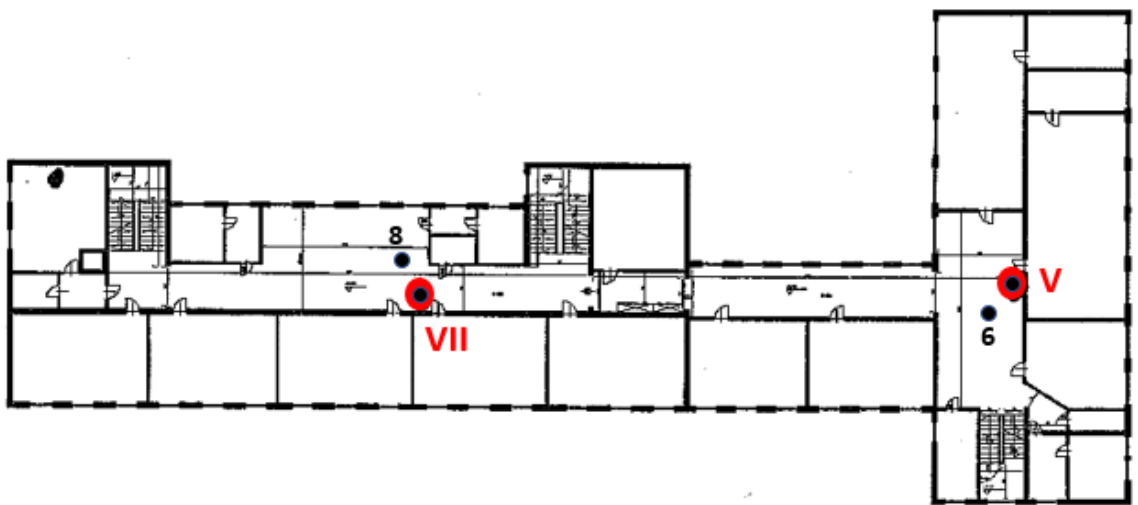
Rys. 1c: Plan rozmieszczenia punktów pomiarowych – II Piętro Liceum, kolorem czerwonym oznaczono lokalizacje punktów dostępowych
