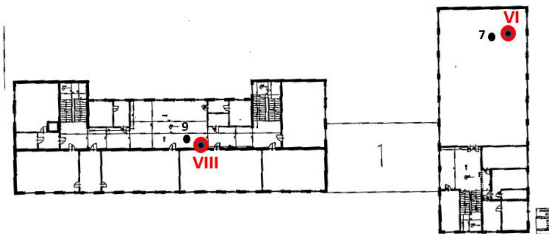
Rys. 1d: Plan rozmieszczenia punktów pomiarowych – III Piętro Liceum
