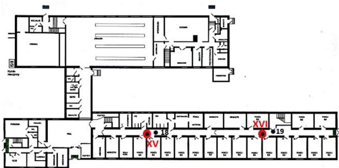
Rys. 1i: Plan rozmieszczenia punktów pomiarowych – Parter Internat
