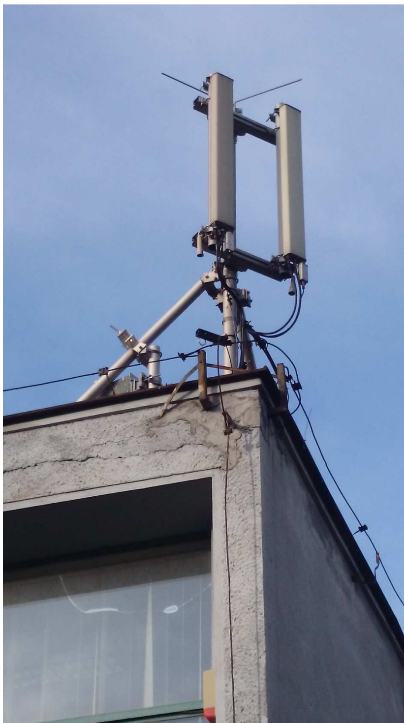
Fot. 3: Widok anten stacji bazowej ID stacji: KRA0222_D zlokalizowanej na dachu budynku użyteczności publicznej w Krakowie przy ul. Kąpielowej 75
