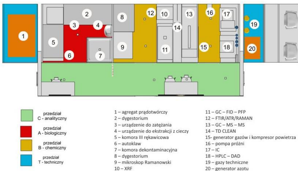
KONCEPCJA ZABUDOWY SAMOCHODU LABORATORIUM DLA WIODĄCYCH GRUP RADIACJI - BILOGII
