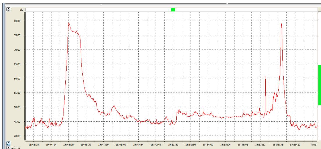
Ryc. 2. Przebieg poziomów dźwięku hałasu kolejowego w funkcji czasu dla przejazdu pociągu towarowego (19:45) i osobowego elektrycznego zespołu trakcyjnego (19:58) w pkt. pom. PR1 – ul. Kolejowa, Poraj, 2013 r.
