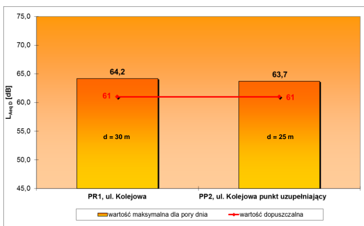
Ryc. 9. Wartości wskaźnika L_{AeqD}^{7d\ max} z okresu 7-miu pór dnia w badanym roku, dla rozpatrywanych punktów referencyjnych oraz ich porównanie z obowiązującymi wartościami poziomów dopuszczalnych, Poraj 2013 rok.
