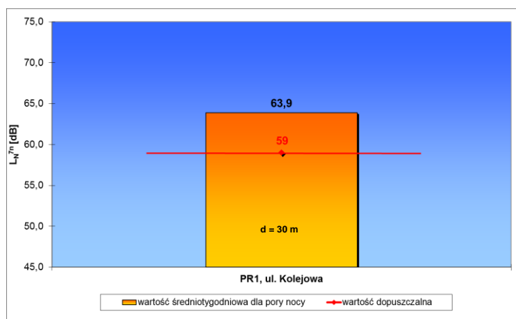
Ryc. 6. Wartości wskaźnika L_N^{7n} poziomów dźwięku dla pory nocy z okresu 7-miu nocy w badanym roku, dla rozpatrywanych punktów referencyjnych oraz ich porównanie z obowiązującymi wartościami poziomów dopuszczalnych, Poraj 2013 rok.
