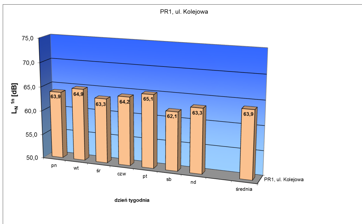
Ryc. 4. Wskaźnik L_N^{1n} (8 h) w [dB]. Zestawienie zmian wskaźnika dla pory nocy ( L_N ) z poszczególnych nocy z 1 tygodniowej sesji pomiarowej wraz z wartością średnią tygodniową, Poraj, 2013 r.
