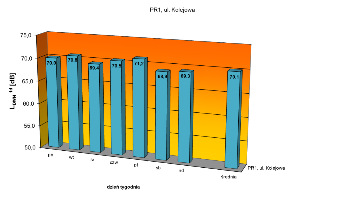
Ryc. 3. Wskaźnik L_{DWN}^{1d} (24 h) w [dB]. Zestawienie zmian wskaźnika dziennie-wieczorno-nocnego ( L_{DWN} ) z poszczególnych dni z 1 tygodniowej sesji pomiarowej wraz z wartością średnią tygodniową, Poraj, 2013 r.
