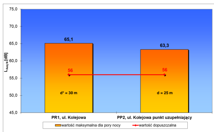
Ryc. 10. Wartości wskaźnika L_{AeqN}^{7n\ max} z okresu 7-miu pór nocy w badanym roku, dla rozpatrywanych punktów referencyjnych oraz ich porównanie z obowiązującymi wartościami poziomów dopuszczalnych, Poraj 2013 rok.
