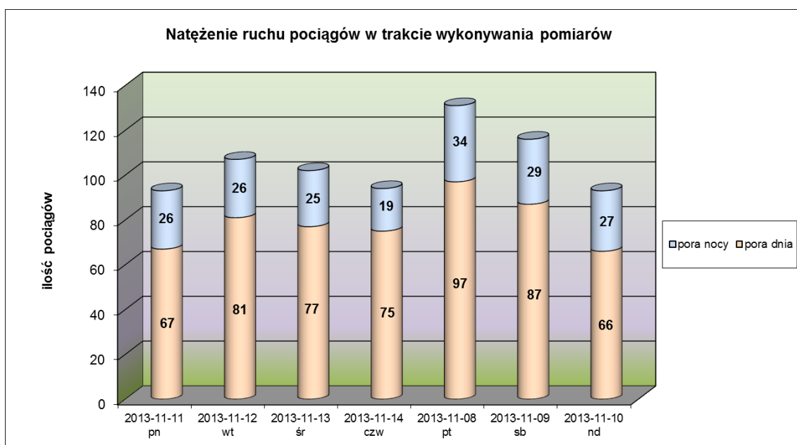
Ryc. 11. Natężenie ruchu pociągów w badanym przekroju pomiarowym, Poraj 2013 rok.
