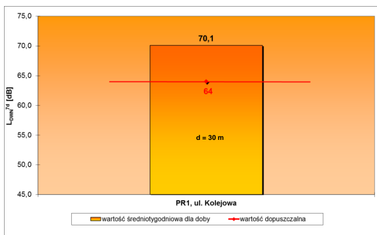
Ryc. 5. Wartości wskaźnika L_{DWN}^{7d} poziomów dźwięku z okresu 7-miu dni w badanym roku, dla rozpatrywanych punktów referencyjnych oraz ich porównanie z obowiązującymi wartościami poziomów dopuszczalnych, Poraj, 2013 rok.
