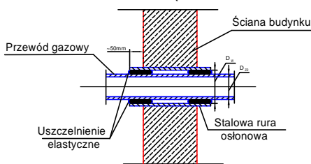
PRZEJŚCIE PRZEWODU GAZOWEGO PRZEZ ŚCIANĘ BUDYNKU
