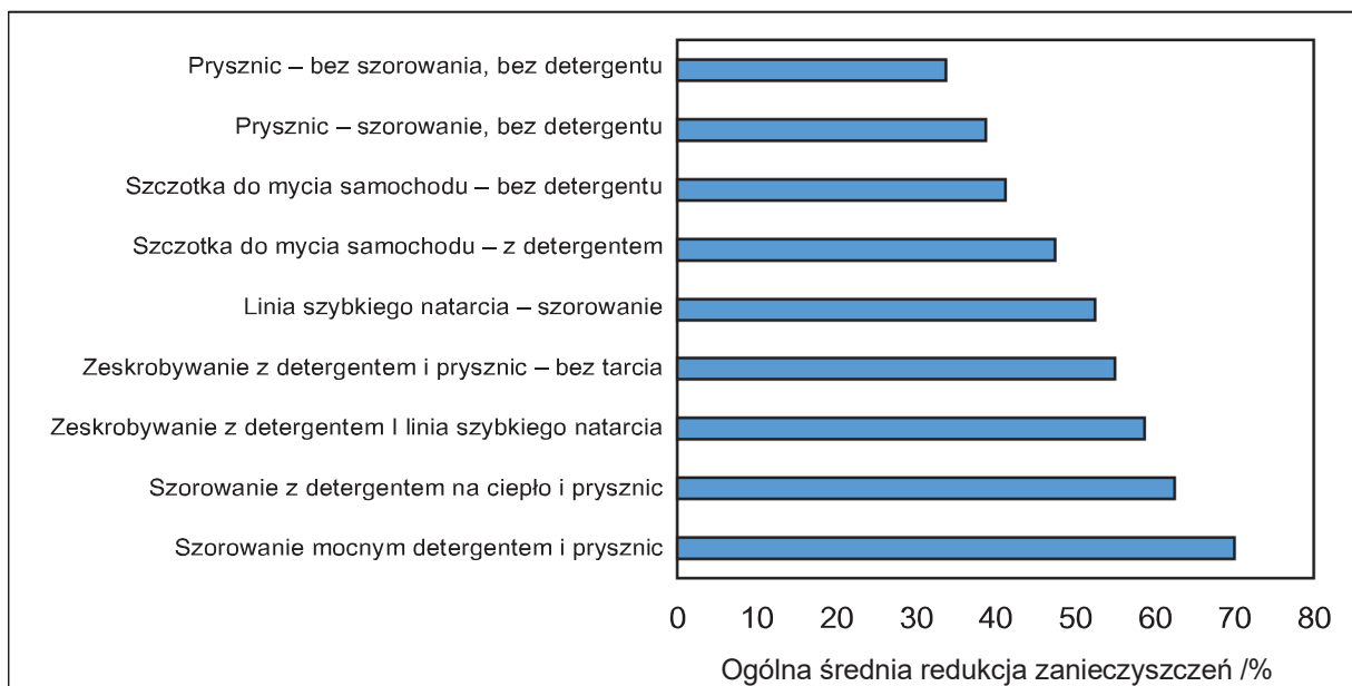
Ilustracja 39 Skuteczność metod odkażania według badań przeprowadzonych przez Home Office Fire and Research and Development Group (1995 – National Operational Guidance (NFCC), 2020)
