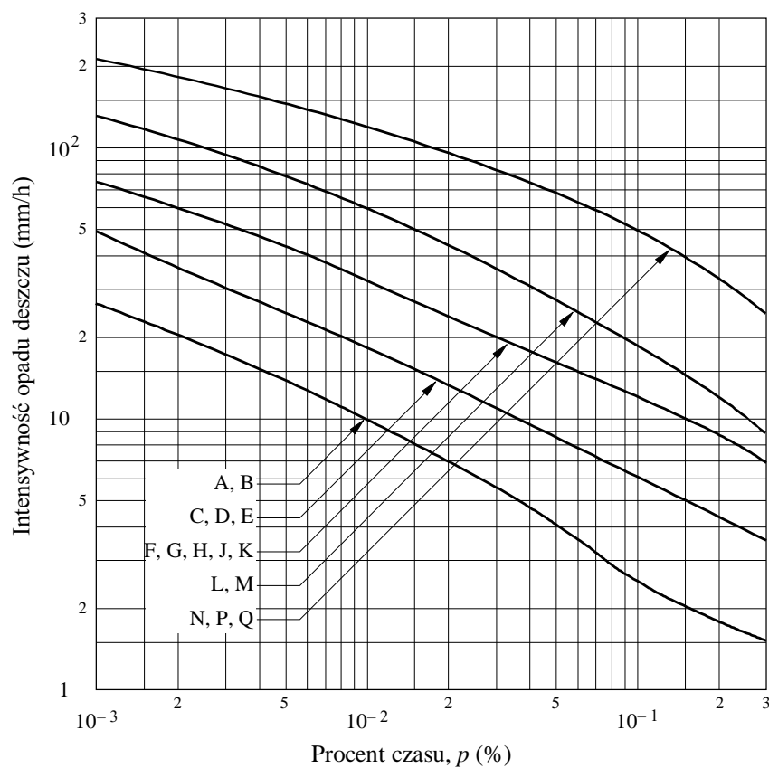
Skonsolidowana dystrybucja intensywności opadu deszczu dla deszczowych stref klimatycznych przedstawionych na Rysunkach 2, 3 i 4
